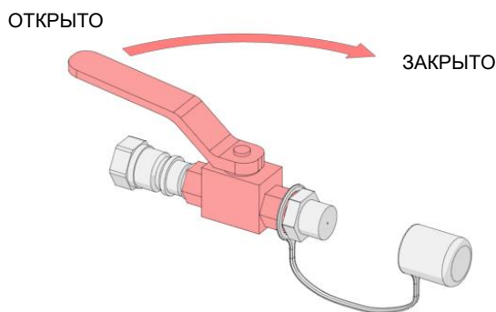
Рисунок 20. Запорный клапан
