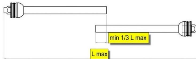
Рисунок 19. Длина крышек шарнирно-телескопического вала
