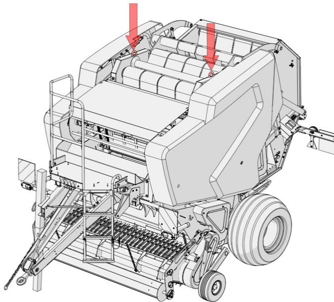
Рисунок 14. Точки крепления подвесного устройства
