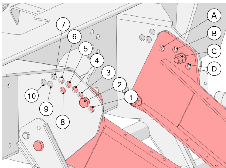
Рисунок 17. Установка высоты дышла
