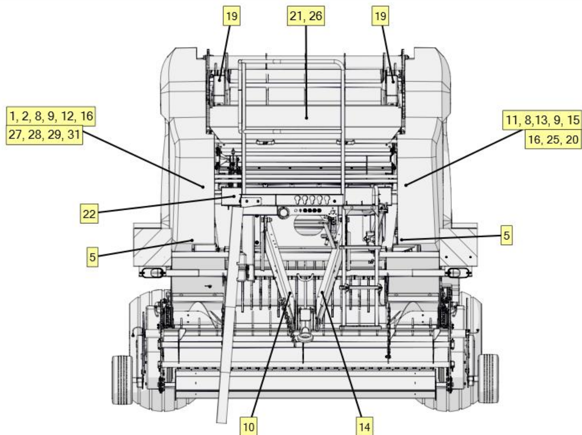
Рисунок 9. Размещение знаков безопасности на машине – спереди
