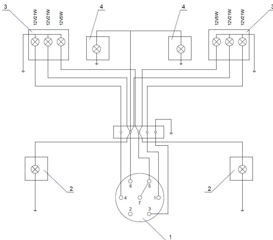
Рисунок 7. Схема электрической системы:
