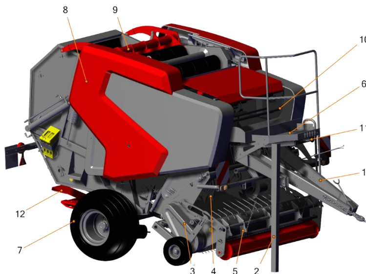
Рисунок 3. Конструкция рулонного пресс-подборщика Z514:
