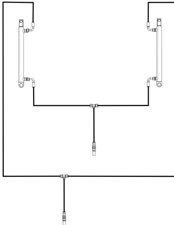
Рисунок 6. Схема гидравлической системы - пол ротора
