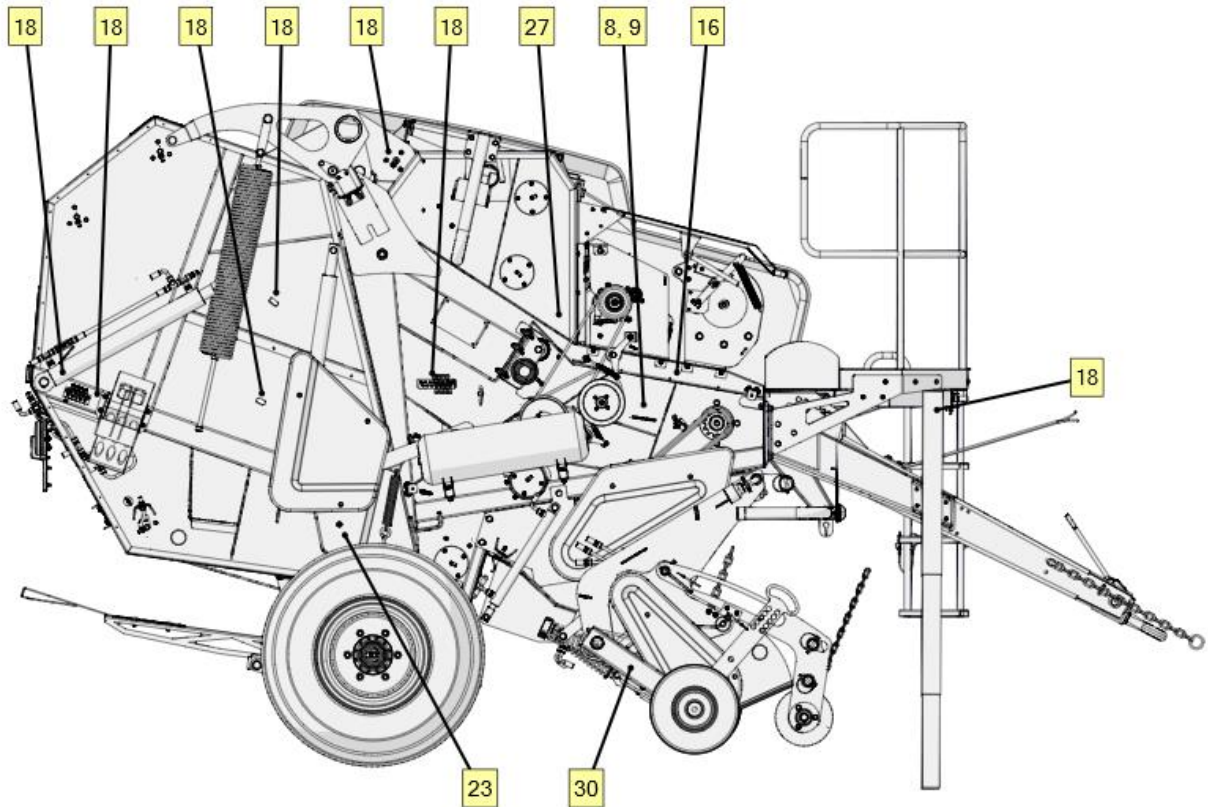
Рисунок 12. Размещение знаков безопасности на машине – правая сторона
