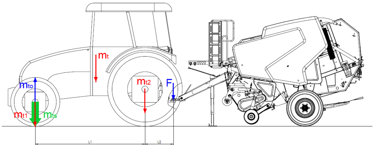
Рисунок 13. Устойчивость состава трактор – пресс-подборщик
