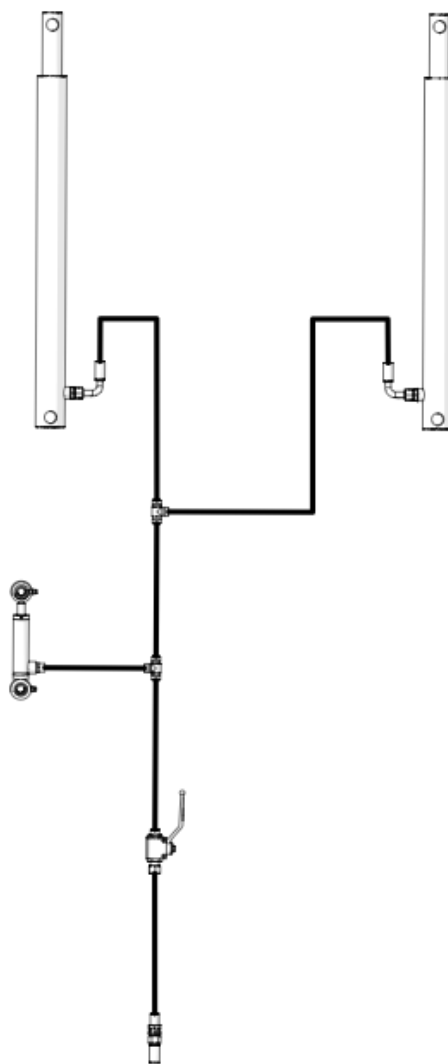
Рисунок 4. Схема гидравлической системы - задняя камерная и механизм обвязки сеткой
