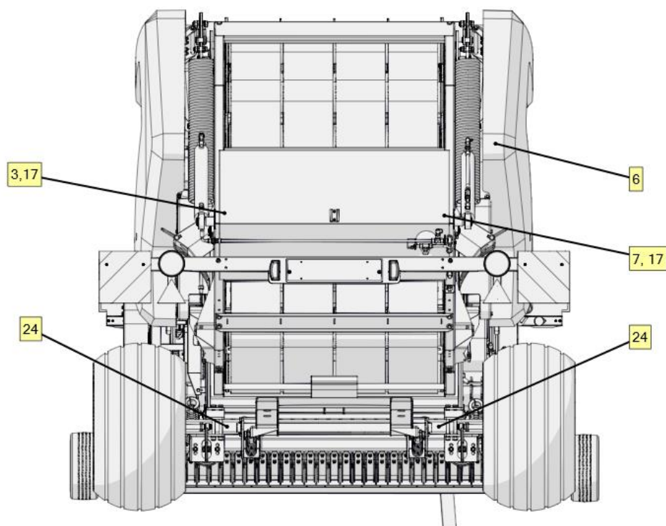
Рисунок 10. Размещение знаков безопасности на машине – сзади
