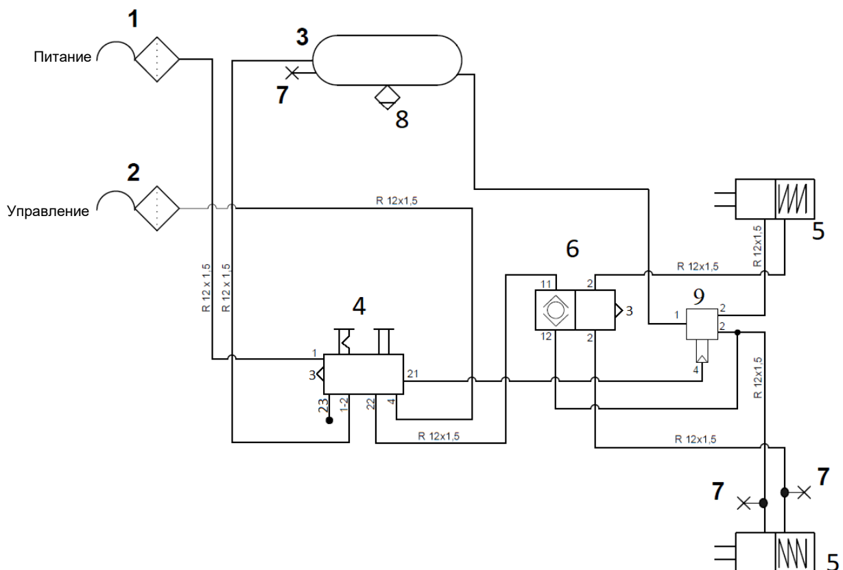
Рисунок 8. Схема тормозной системы:
