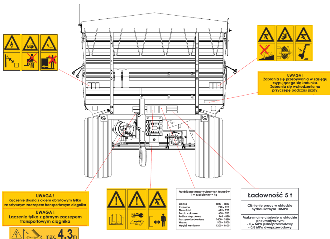
Rysunek 4. Rozmieszczenie piktogramów na ścianach przyczepy – przód
