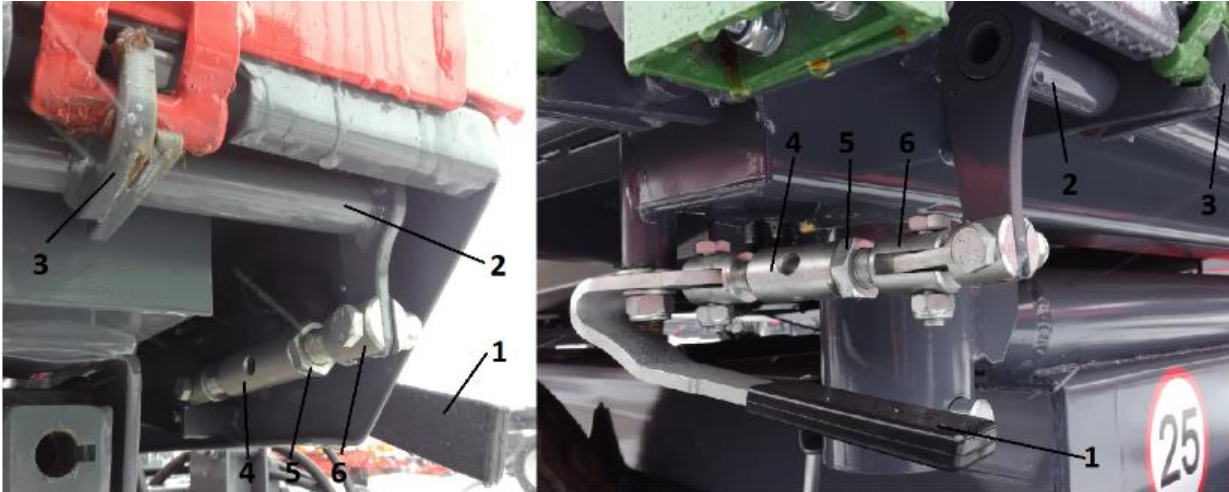
Rysunek 16. Zamki ścian skrzyni ładunkowej:
