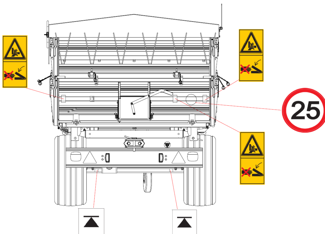
Rysunek 5. Rozmieszczenie piktogramów na ścianach przyczepy - tył
