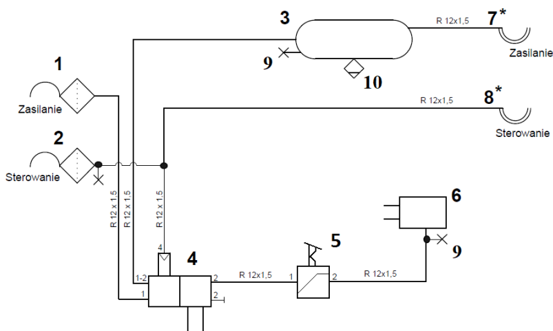
Rysunek 13. Schemat pneumatycznej instalacji hamulcowej dwuprzewodowej
