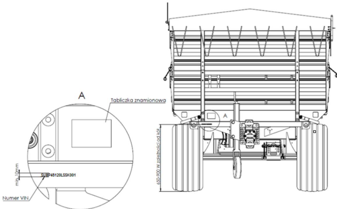
Rysunek 1. Umieszczenie tabliczki znamionowej
