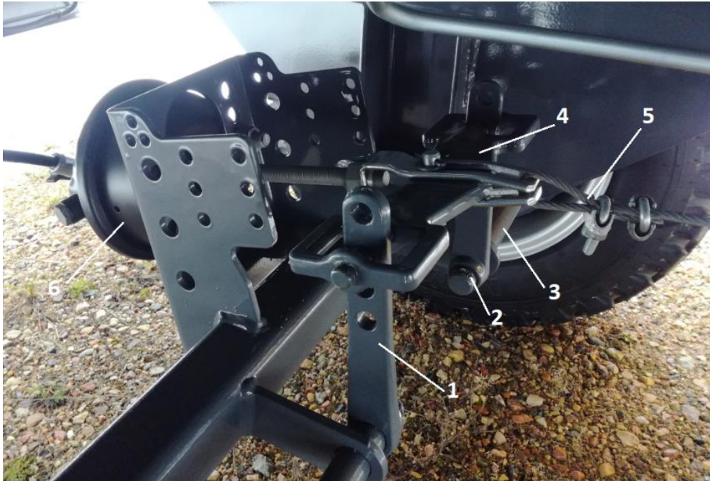
Rysunek 17. Elementy układu hamulcowego:
