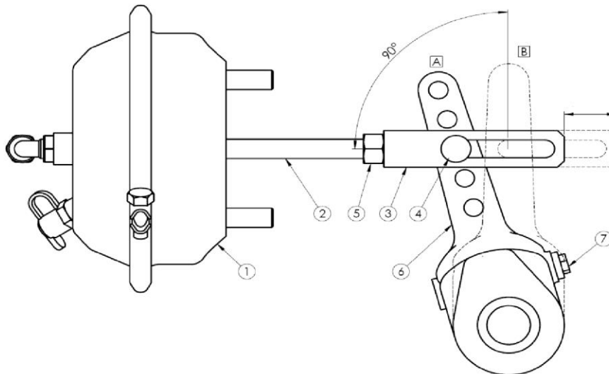
Abbildung 43. Einstellung der Betriebsbremse
