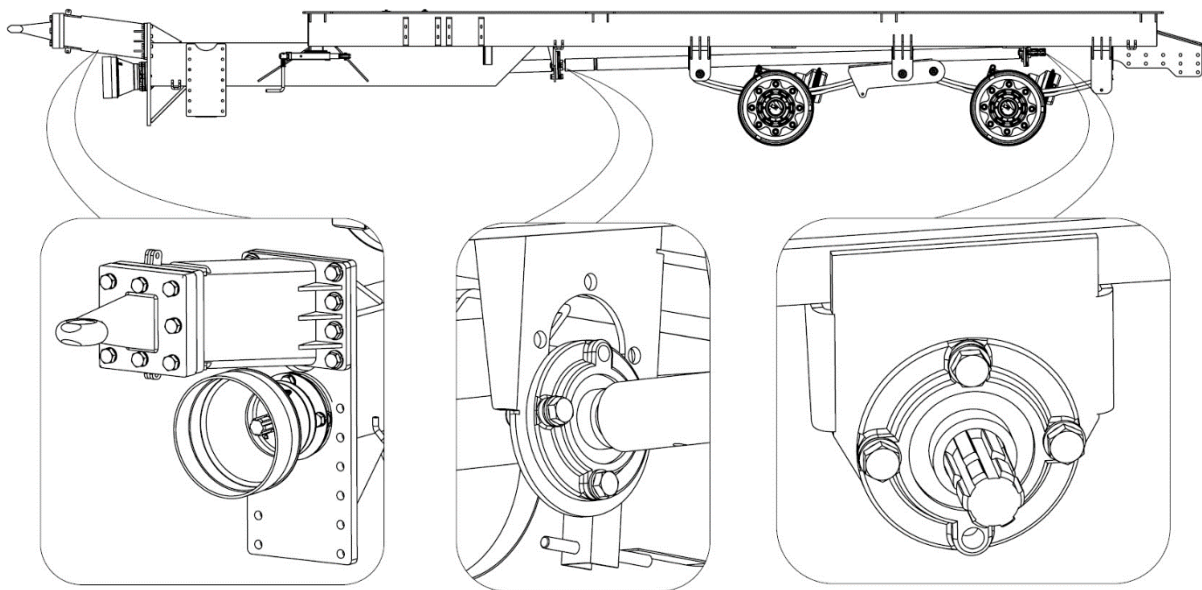
Abbildung 17. Position der Anhängerkupplung, die zum Anschluss an den Unterlenker des Schleppers geeignet ist
