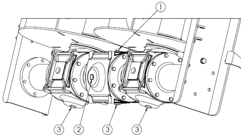
Abbildung 30. Ölstands-Kontrollpunkte des Rollbodengetriebes. 1 - Ölfüllöffnung (Entlüftung), 2 - Ölstandschauflas, 3 – Ablassschraube
