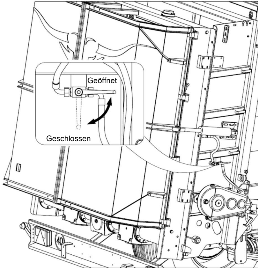
Abbildung 25. Hydraulikventil zur Verriegelung der Adapterabdeckung
