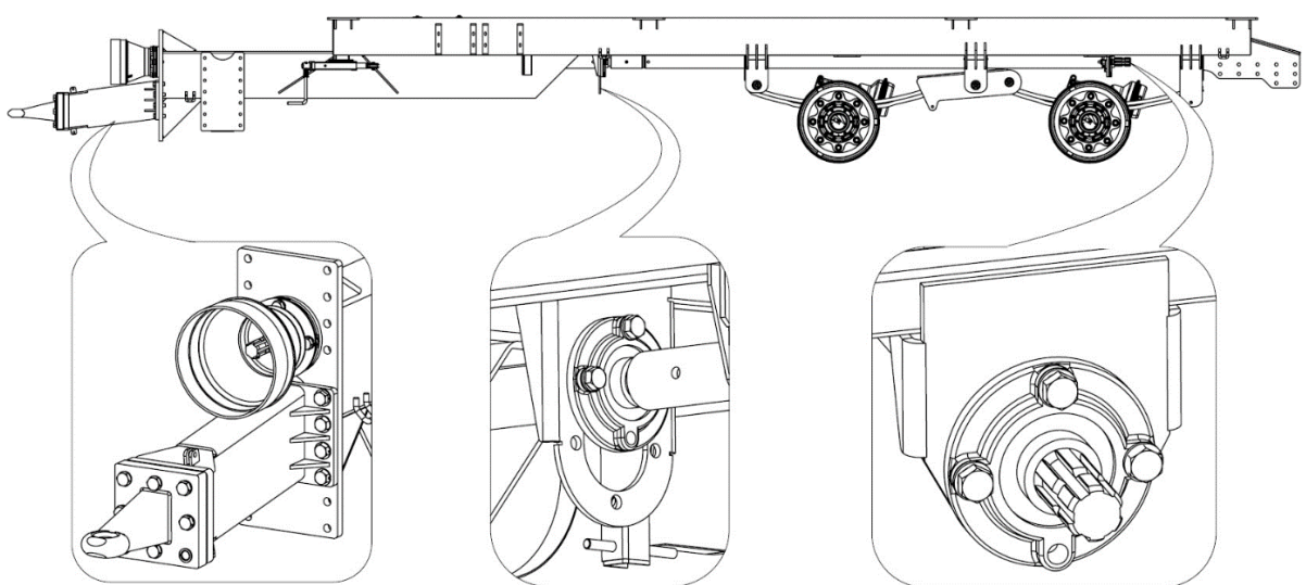
Abbildung 18. Position der Anhängerkupplung, die zum Anschluss an den Oberlenker des Schleppers geeignet ist
