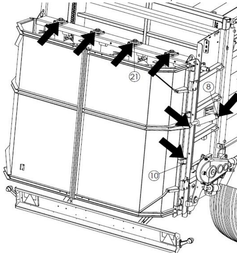
Abbildung 36. Schmierstellen des Streuers (horizontaler Scheibenadapter mit Zweifach-Rotor)
