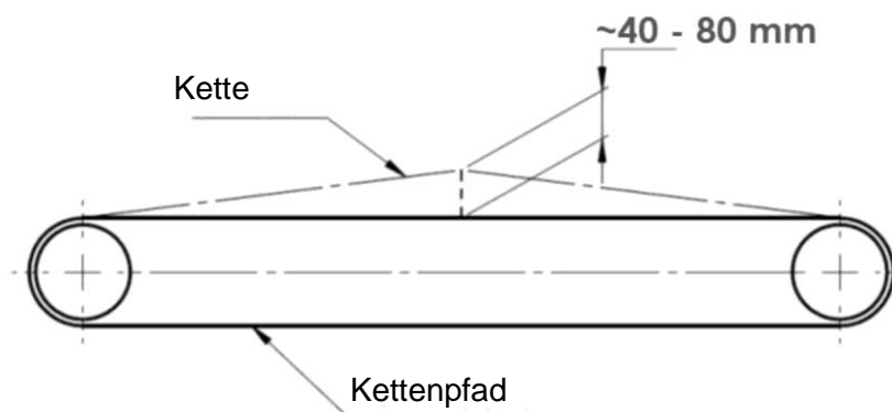
Abbildung 28. Überprüfung der Kettenspannung im Streuer
