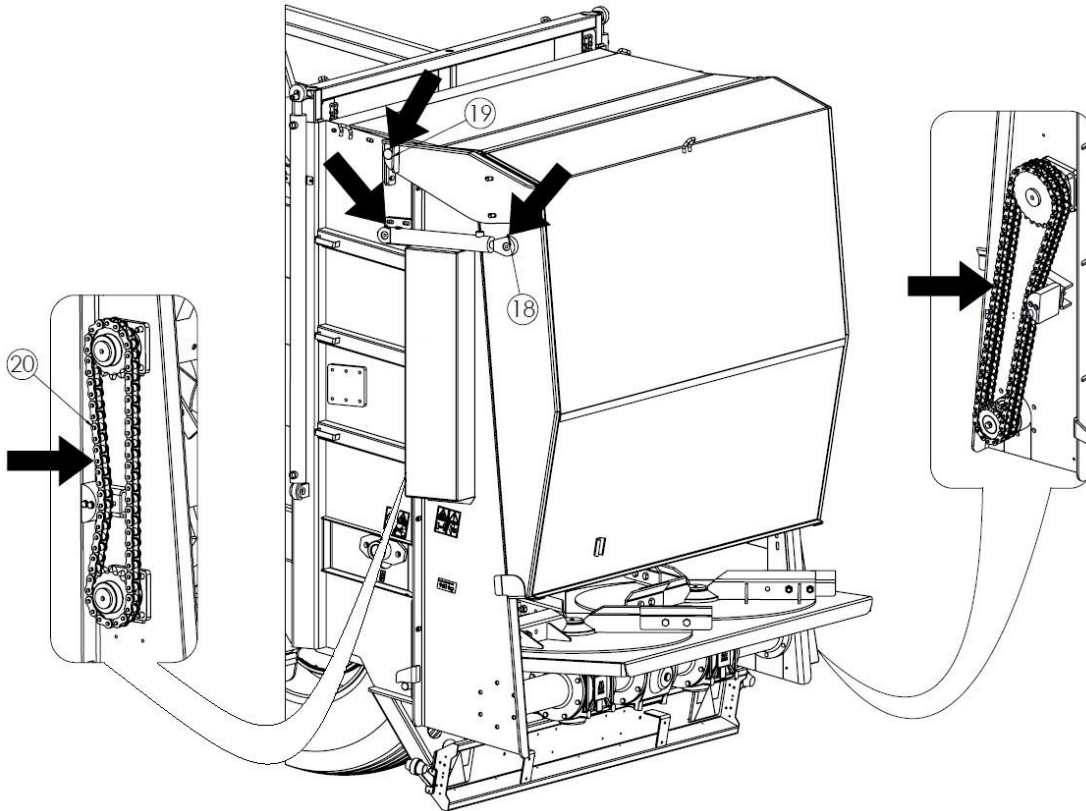
Abbildung 36. Schmierstellen des Streuers (horizontaler Scheibenadapter mit Zweifach-Rotor)
