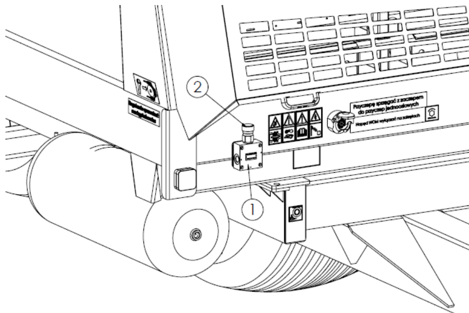
Abbildung 24. Einstellung der Rollbodengeschwindigkeit 1 - Ölmenge, 2 - Drehknopf des Reglers
