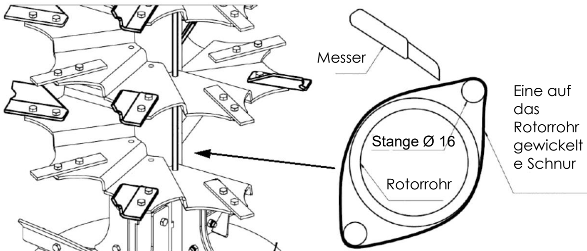
Abbildung 46. Entfernen von aufgewickelten Schnüren, Netzen
