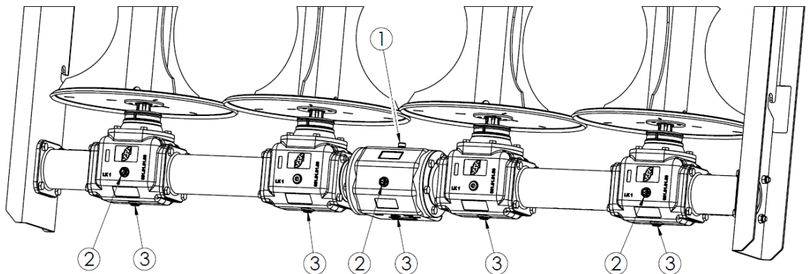
Abbildung 31. Ölstands-Kontrollpunkte des Getriebes des vertikalen Streuadapters mit Zweifach-Rotor und des horizontalen Scheibenadapters mit Zweifach-Rotor 1 - Ölfüllöffnung (Entlüftung), 2 - Ölstandschauflas, 3 – Ablassschraube
