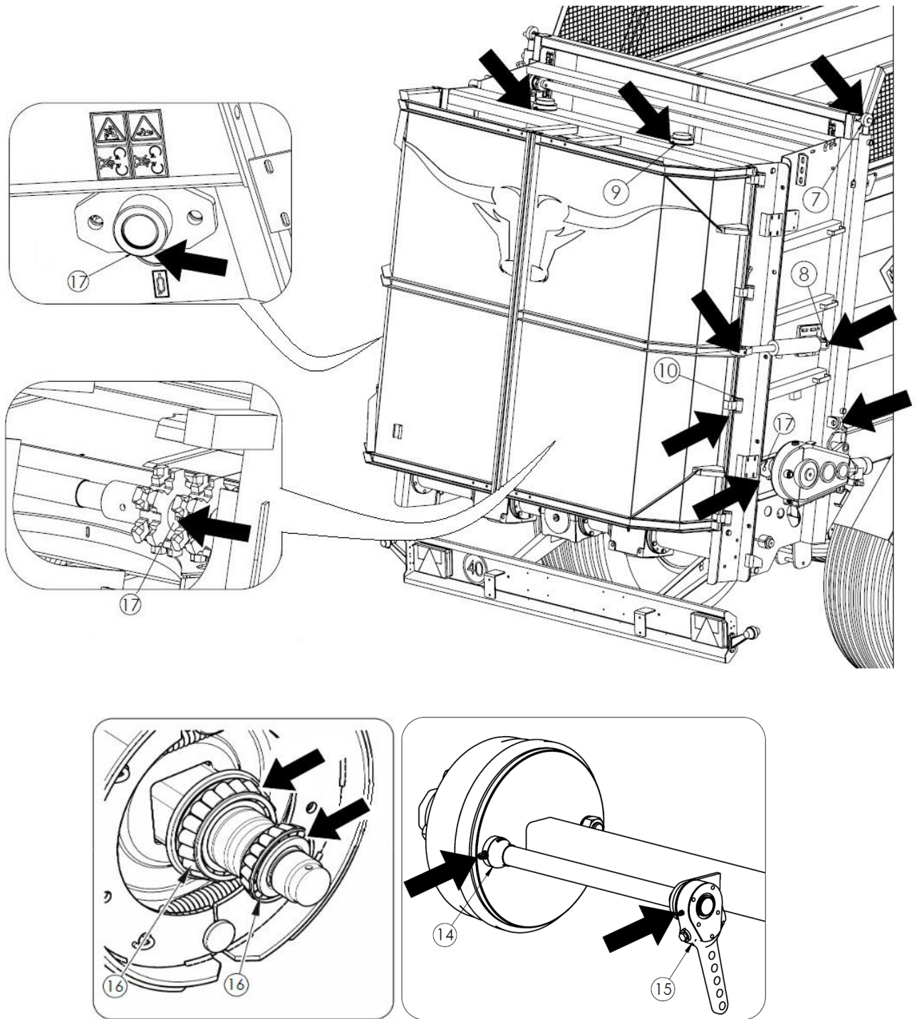
Abbildung 35. Schmierstellen des Streuers
