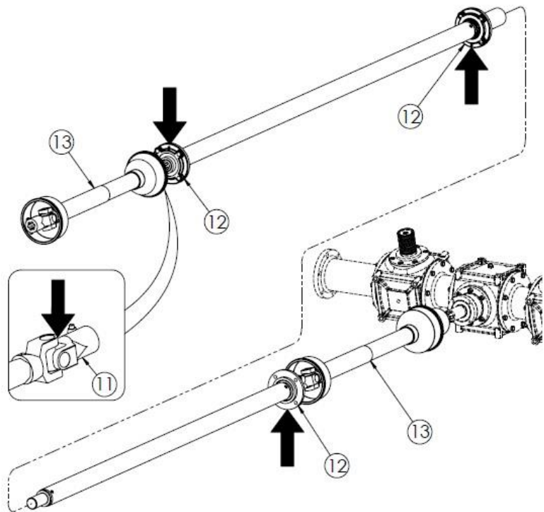
Abbildung 34. Schmierstellen des Streuers
