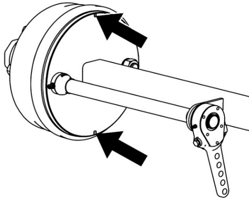
Abbildung 42. Verschleißkontrolle des Bremsbelags
