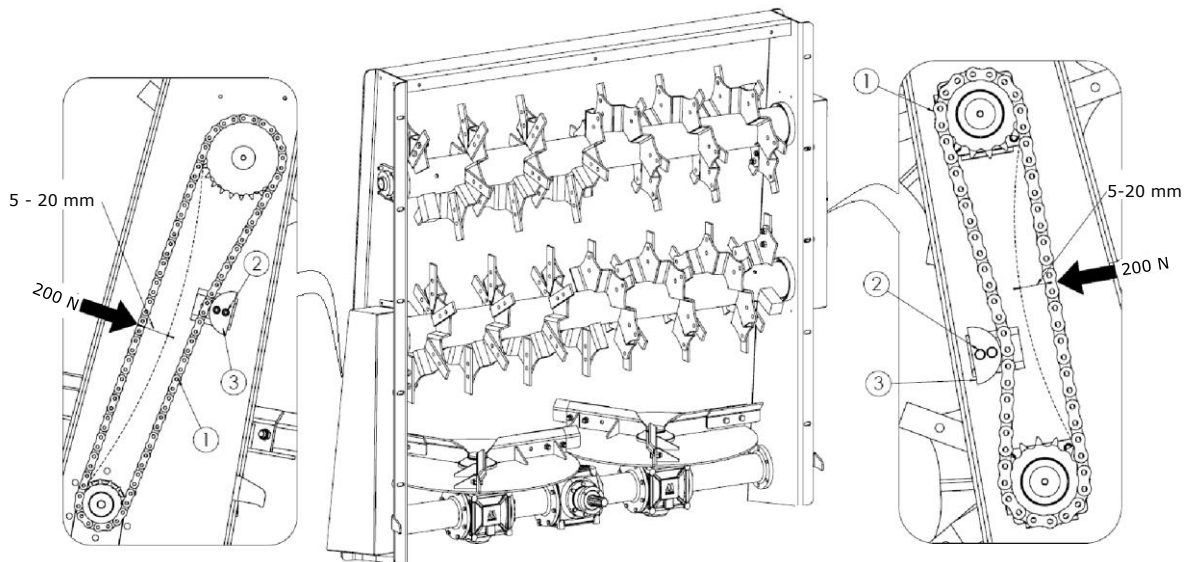
Abbildung 29. Spannen der Adapterketten
