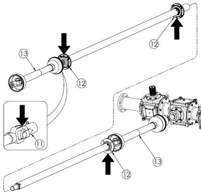
Рисунок 34. Точки смазки навозоразбрасывателя
