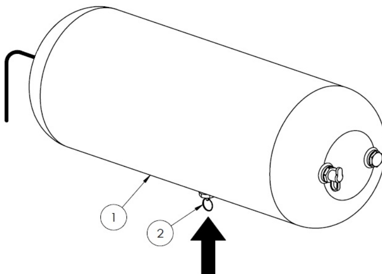
Рисунок 40. Слив воды из ресивера: 1 - ресивер, 2 - клапан водоотвода
