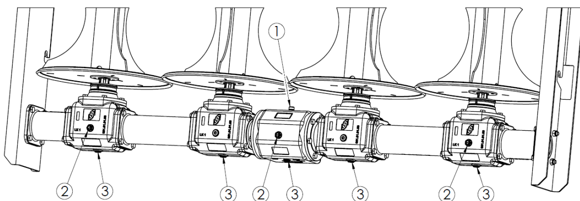
Рисунок 31. Точки контроля уровня масла редуктора двухроторного вертикального адаптера и двухроторного горизонтального дискового адаптера 1 - заливное отверстие (сапун), 2 - контрольный глазок, 3 - сливные пробки
