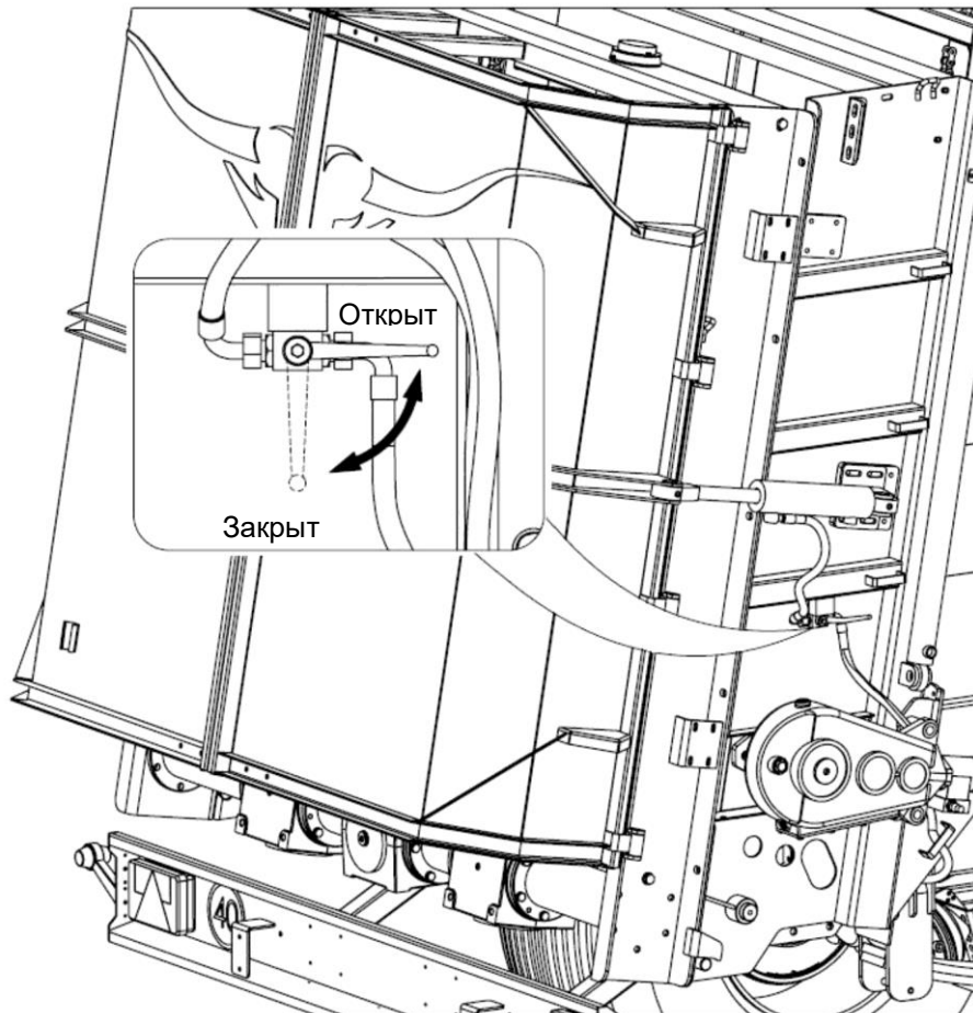
Рисунок 25. Гидравлический клапан для блокировки крышки адаптера
