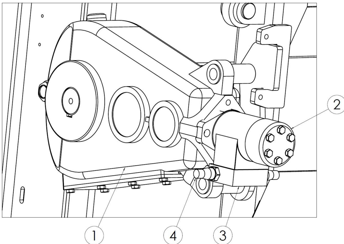
Рисунок 26. Привод напольного конвейера
