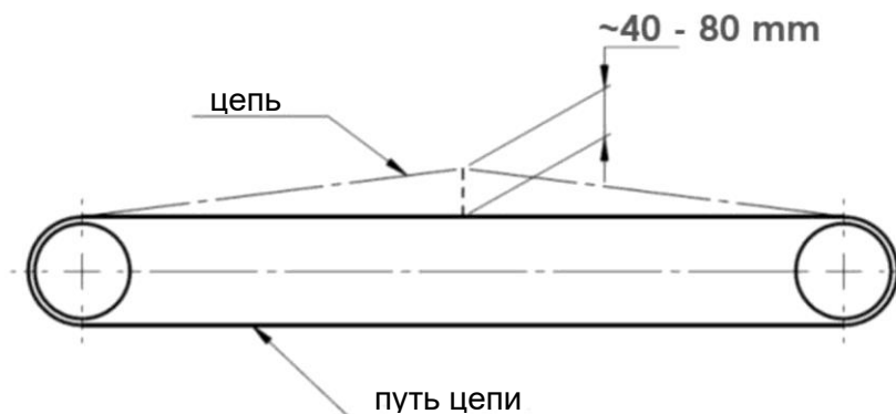
Рисунок 28. Проверка натяжения цепи в навозоразбрасывателе
