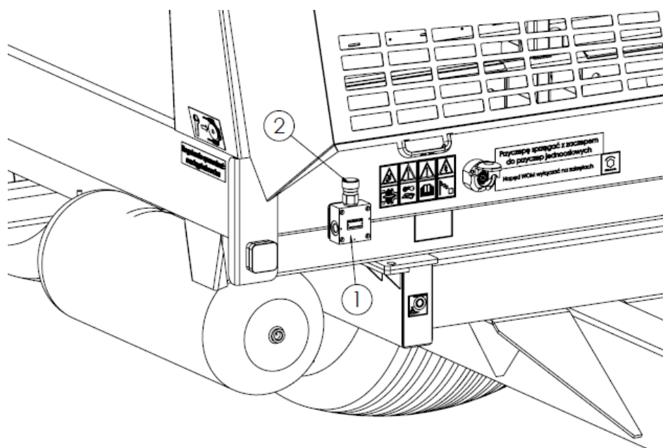
Рисунок 24. Регулировка скорости перемещения напольного конвейера 1 - регулятор потока масла, 2 - ручка регулятора
