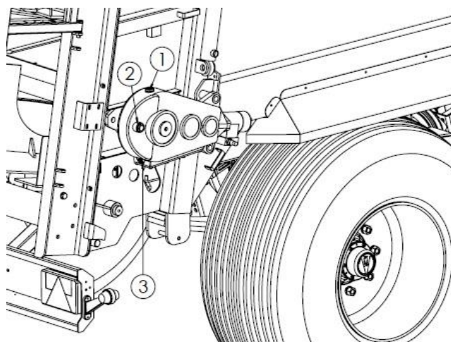
Рисунок 30. Точки контроля уровня масла редуктора напольного конвейера 1 - заливное отверстие (сапун), 2 - контрольный глазок, 3 - сливная пробка
