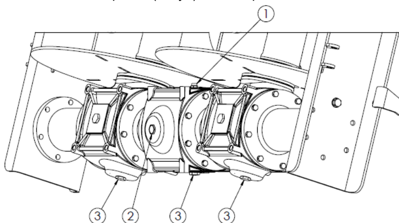
Рисунок 31. Точки контроля уровня масла редуктора двухроторного вертикального адаптера и двухроторного горизонтального дискового адаптера 1 - заливное отверстие (сапун), 2 - контрольный глазок, 3 - сливные пробки
