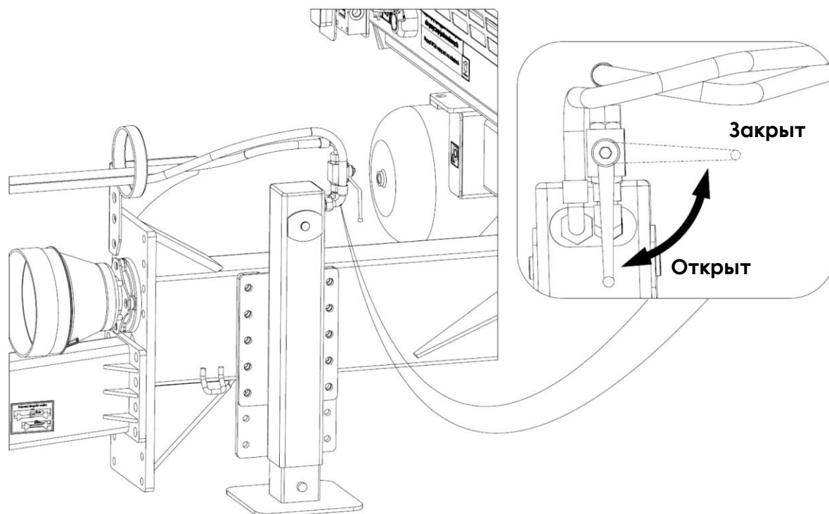
Рисунок 20. Гидравлический клапан управления (отключения) гидравлической пятой
