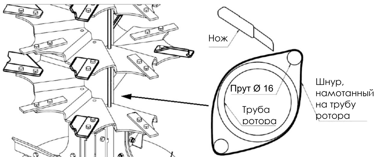
Рисунок 46. Очистка намотанных шнуров, сеток
