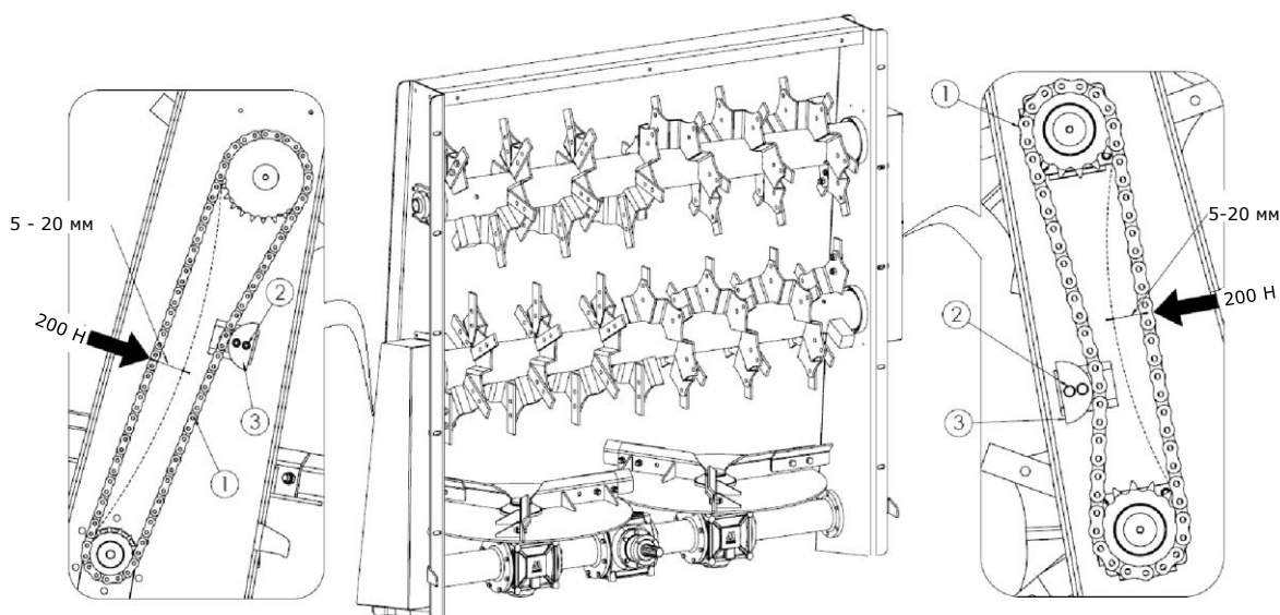
Рисунок 29. Натяжение цепей адаптера
