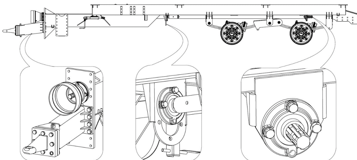
Рисунок 18. Положение сцепки, пригодной для соединения с верхней сцепкой трактора
