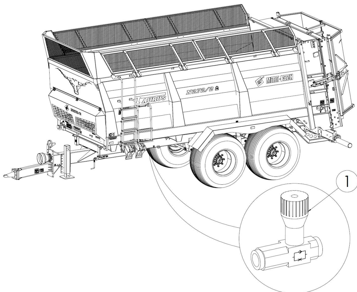
Рисунок 33. Регулятор открытия заслонки
