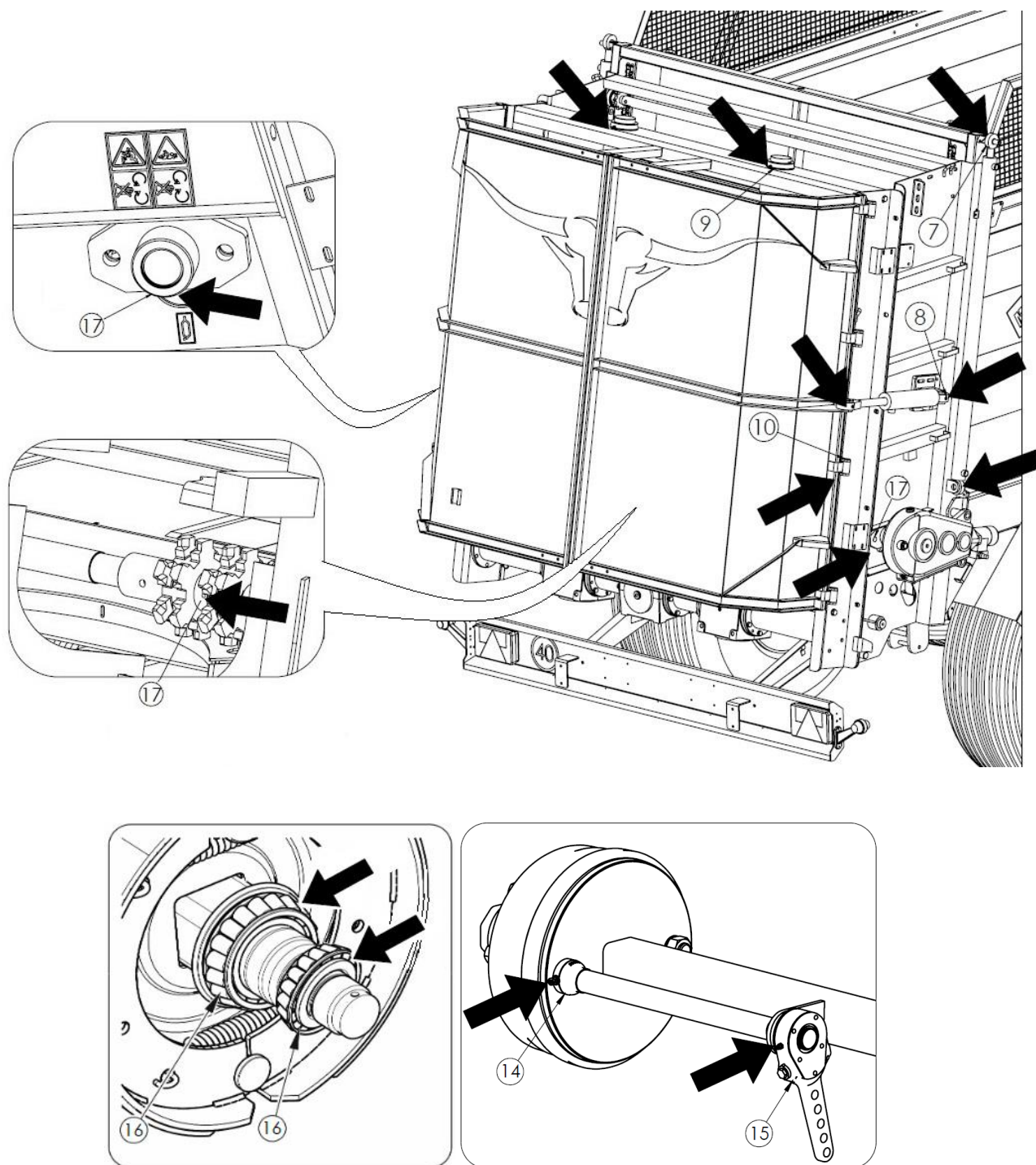
Рисунок 35. Точки смазки навозоразбрасывателя
