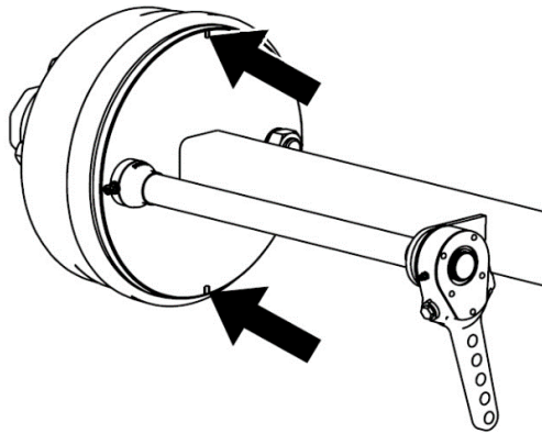
Рисунок 42. Проверка износа накладок тормозных колодок
