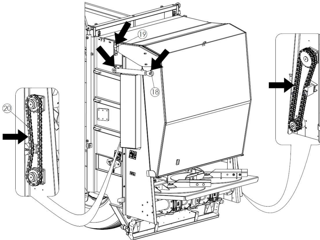
Рисунок 36. Точки смазки навозоразбрасывателя (двухроторный дисковый горизонтальный адаптер)
