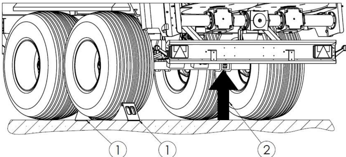
Рисунок 44. Точки установки домкратов 1 - упоры, 2 – домкрат
