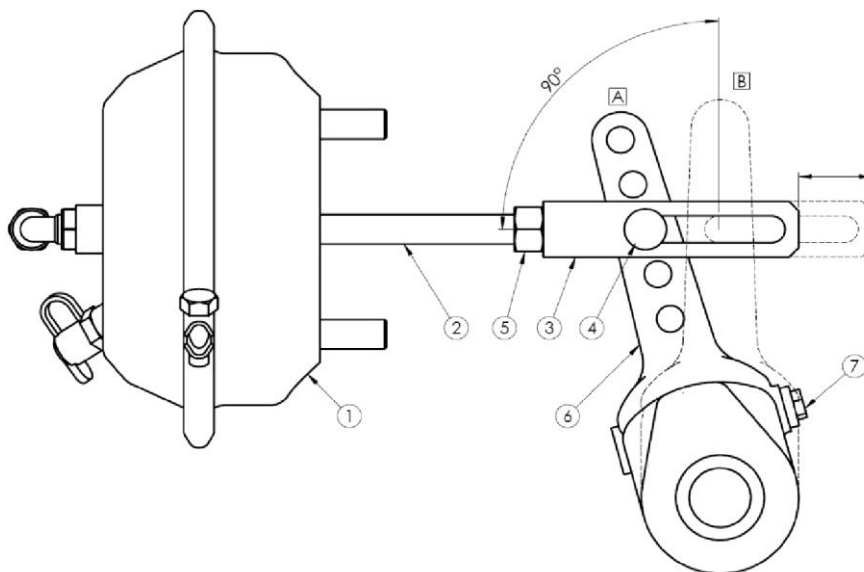
Рисунок 43. Регулировка рабочего тормоза
