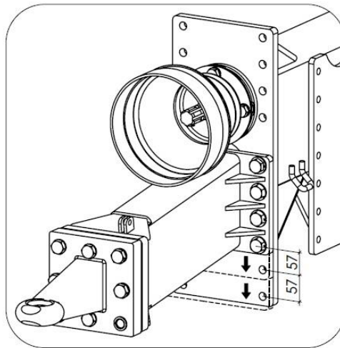
Рисунок 19. Регулировка высоты сцепного устройства
