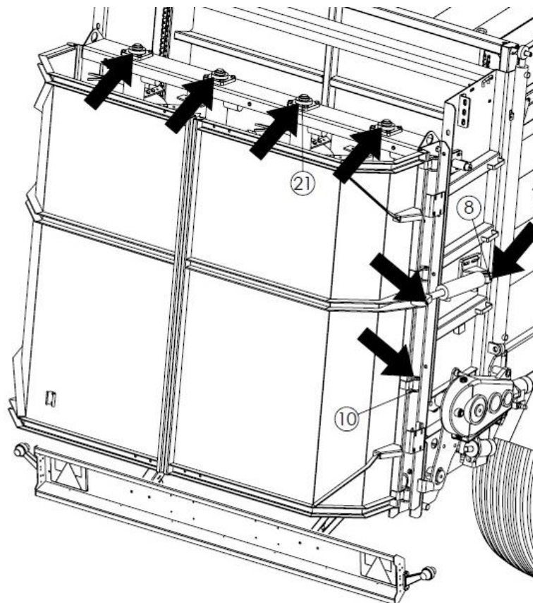
Рисунок 37. Точки смазки навозоразбрасывателя (четырёхроторный вертикальный адаптер)
