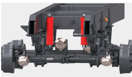
Stabilizacja hydrauliczna osi
