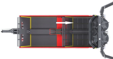
System zsuwający nadający się również do ciężkich ładunków
