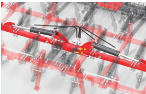
U487 NOVALIS TRIO 420 - rama składana hydraulicznie
