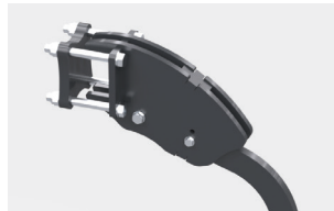
Zabezpieczenie śrubowe elementów roboczych
