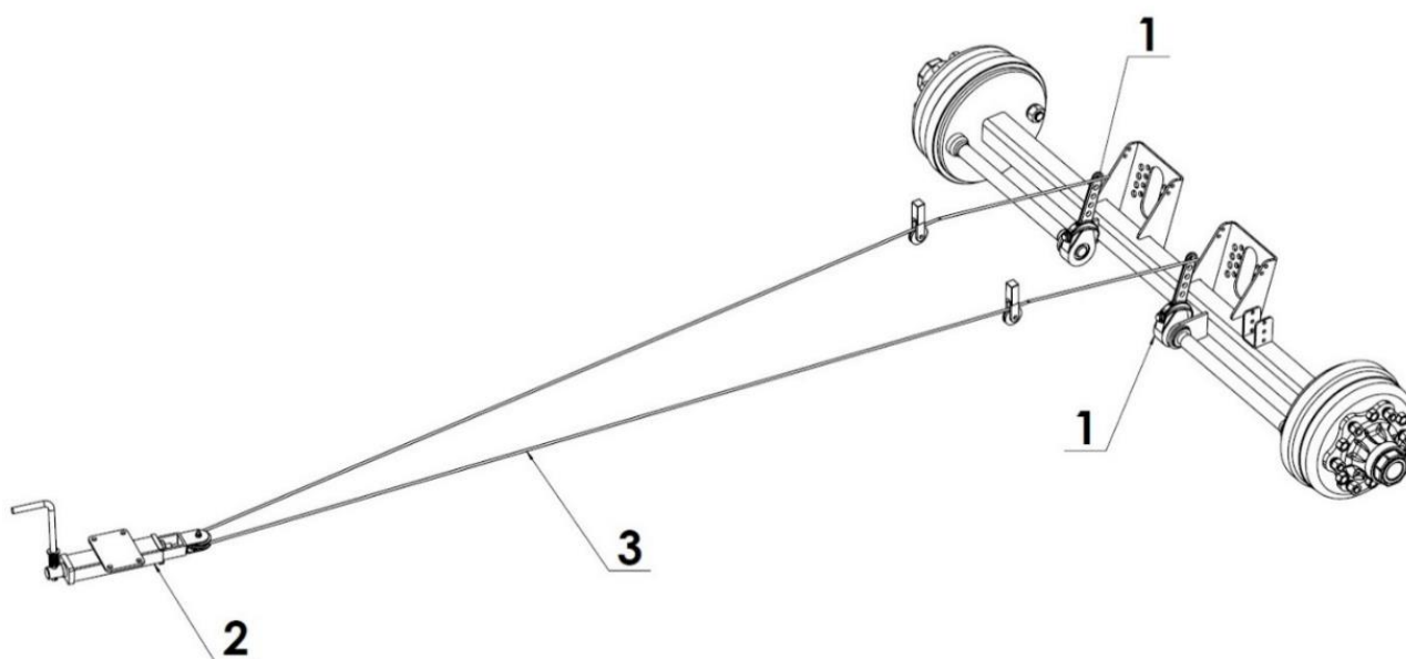
Rysunek 12. Hamulec postojowy:
