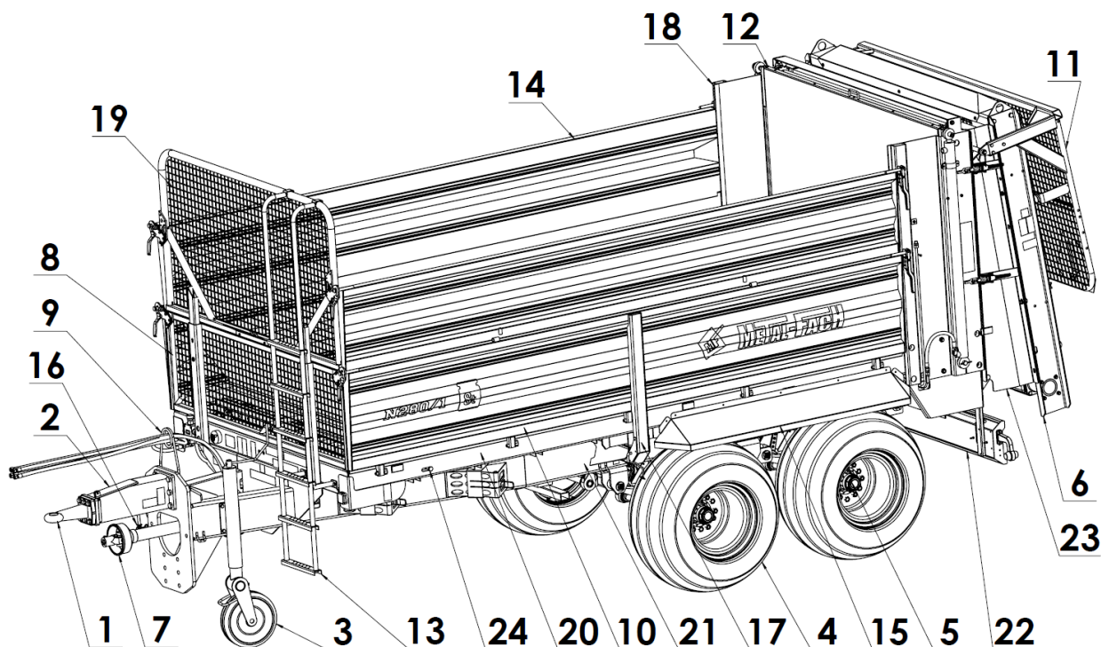
Rysunek 4. Ogólna budowa rozrzutnika obornika:
