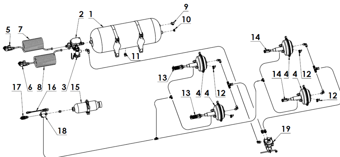
Rysunek 11. Instalacja hamulcowa pneumatyczno – hydrauliczna z zaworem ALB:
