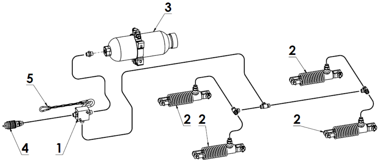
Rysunek 9. Instalacja hamulcowa hydrauliczna 1-przewodowa:
