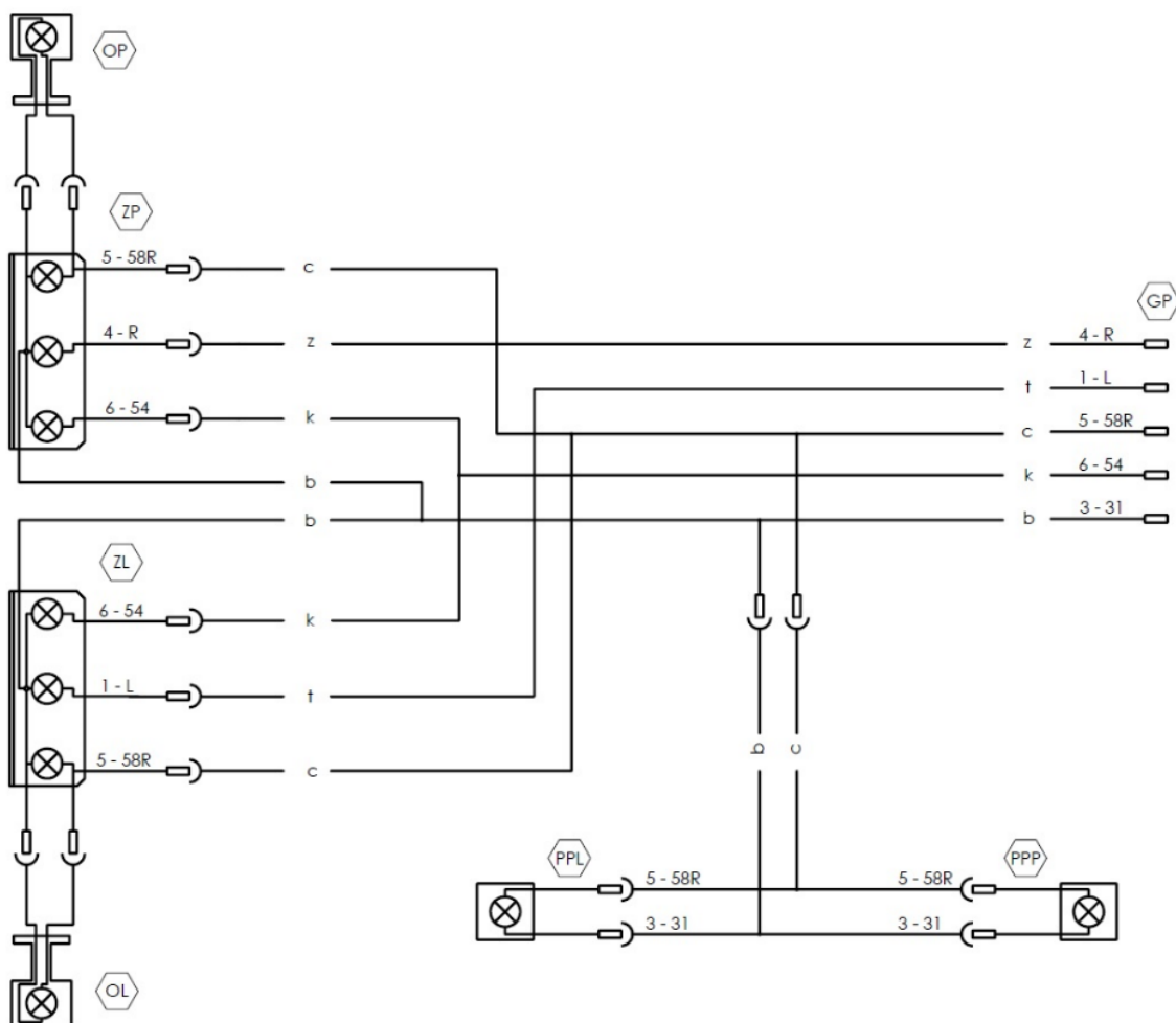
Rysunek 13. Schemat instalacji elektrycznej
