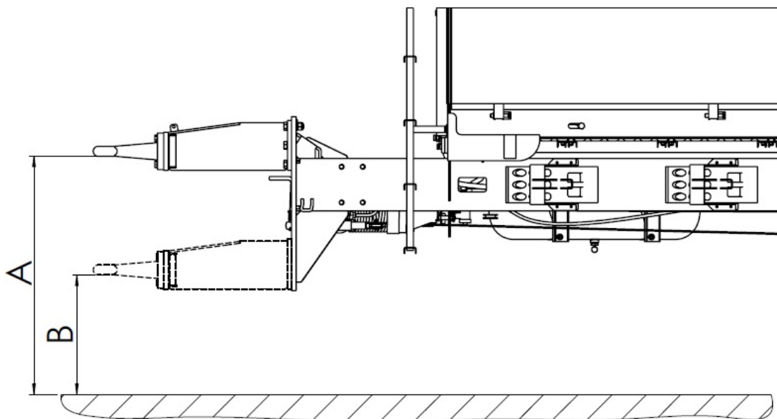
Rysunek 16. Położenie dyszla względem podłoża
