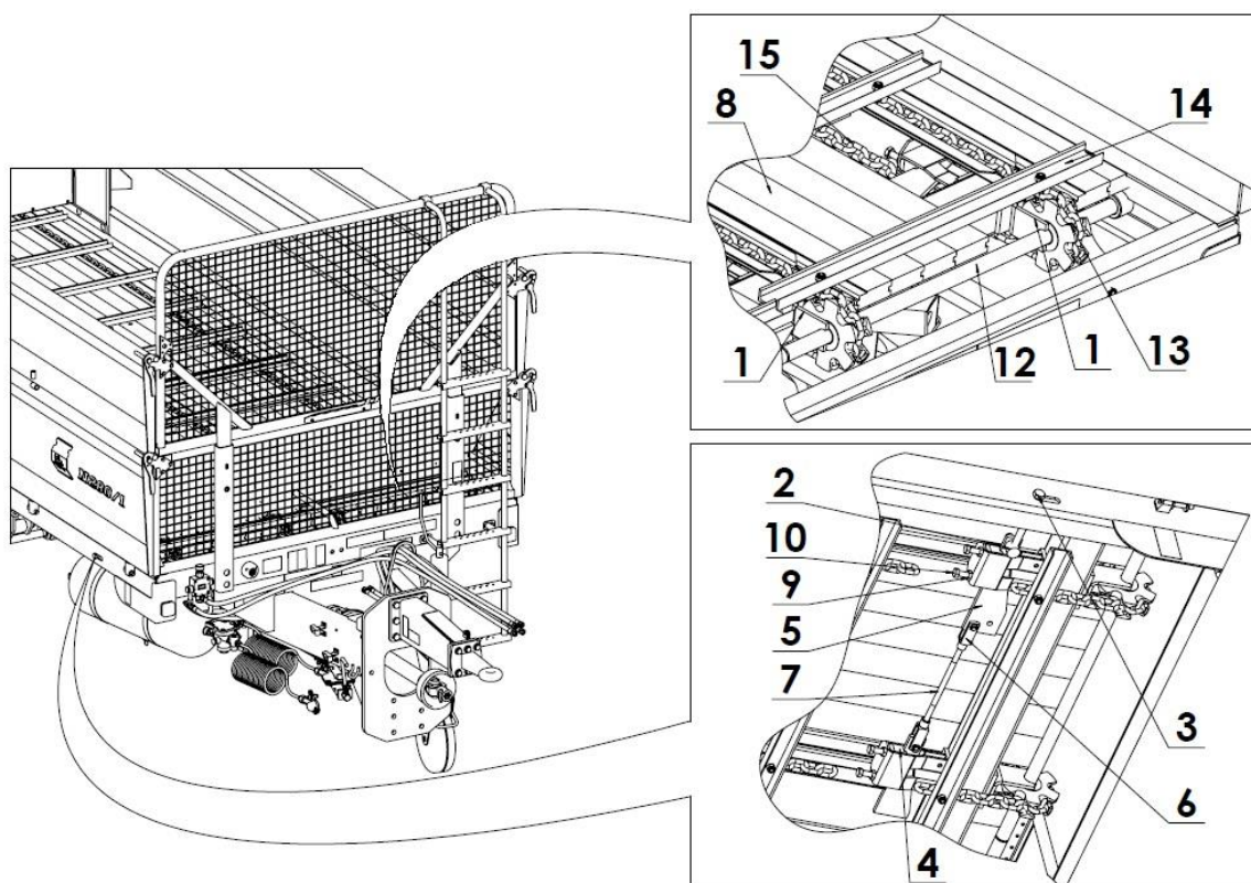
Rysunek 19. Napinanie łańcuchów przenośnika podłogowego:
