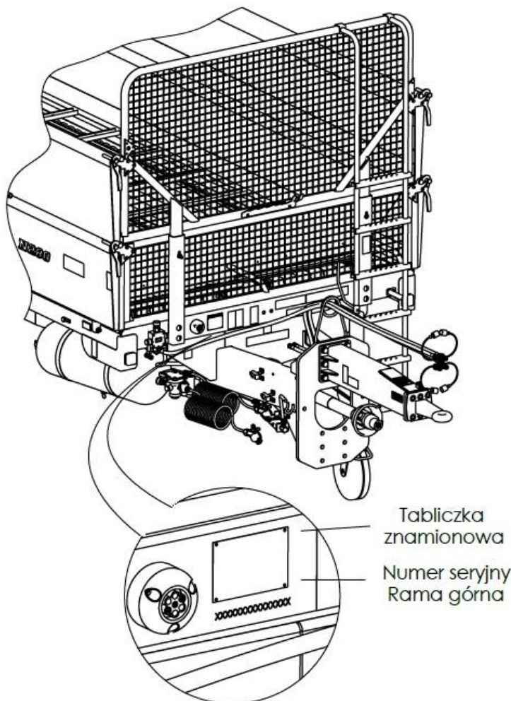
Rysunek 1. Położenie tabliczki znamionowej i numeru seryjnego
