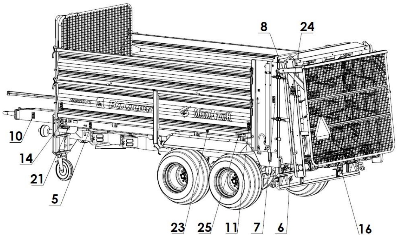
Rysunek 3. Rozmieszczenie naklejek ostrzegawczych i informacyjnych
