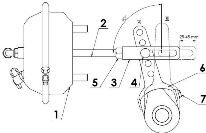
Rysunek 32. Regulacja hamulca zasadniczego:
