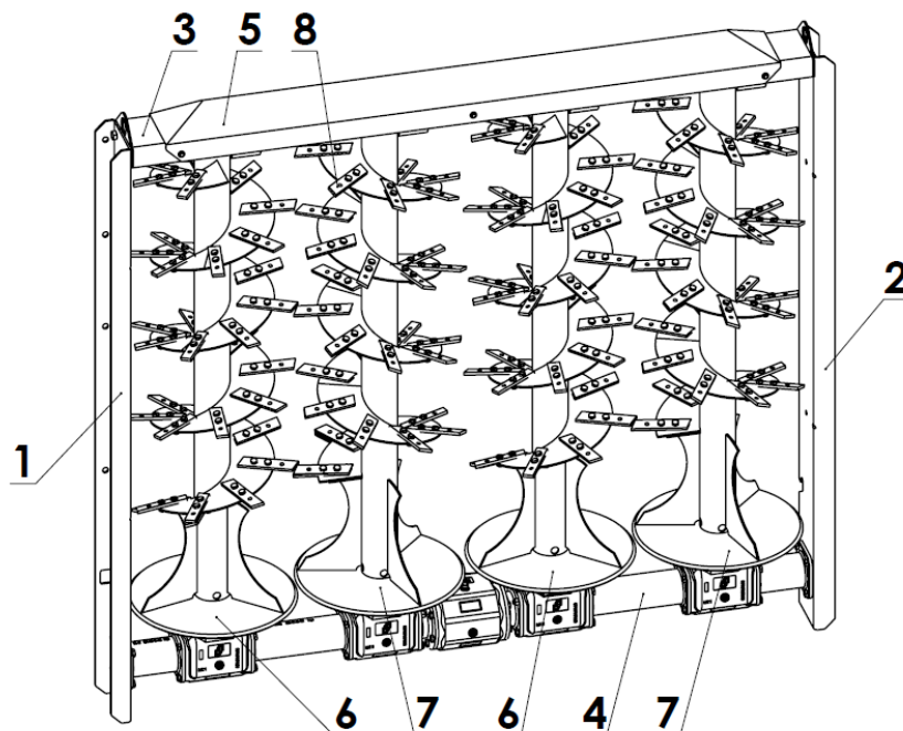
Rysunek 5. Adapter pionowy 2-wirnikowy
