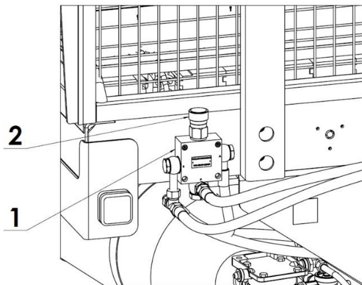
Rysunek 17. Regulacja prędkości przesuwu przenośnika podłogowego: 1 - regulator przyływu oleju, 2 - pokrętło regulatora
