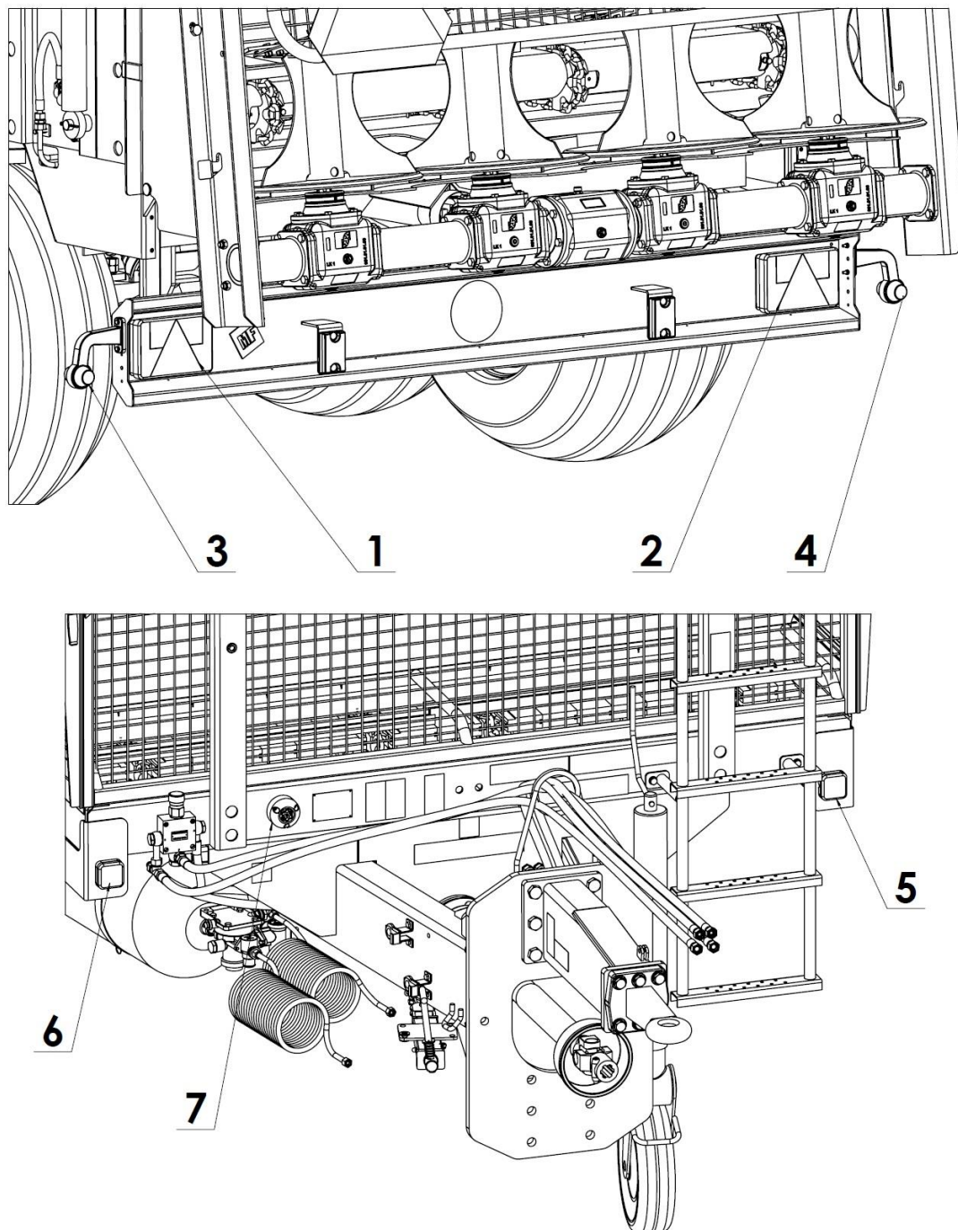
Rysunek 14. Rozmieszczenie elementów instalacji elektrycznej:
