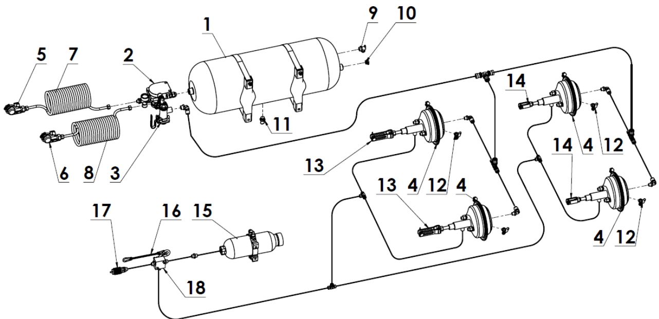
Rysunek 10. Układ hamulcowy hydrauliczno-pneumatyczny:
