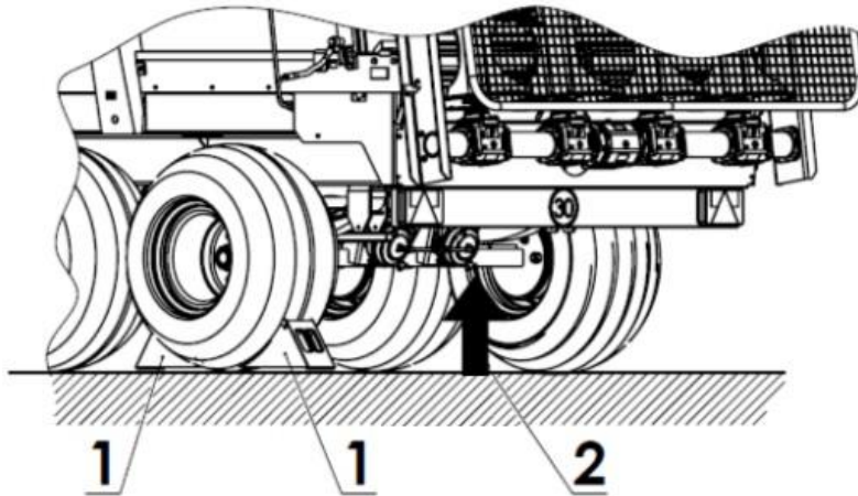
Rysunek 33. Punkty przyłożenia podnośników: 1 - kliny, 2 - podnośnik
