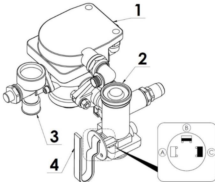
Rysunek 8. Zawór sterujący i regulator siły hamowania hamulców pneumatycznych 2-przewodowych:
