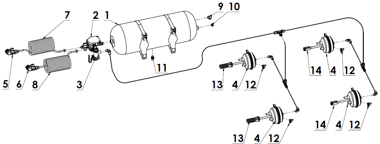
Rysunek 6. Instalacja hamulcowa pneumatyczna 2-przewodowa:
