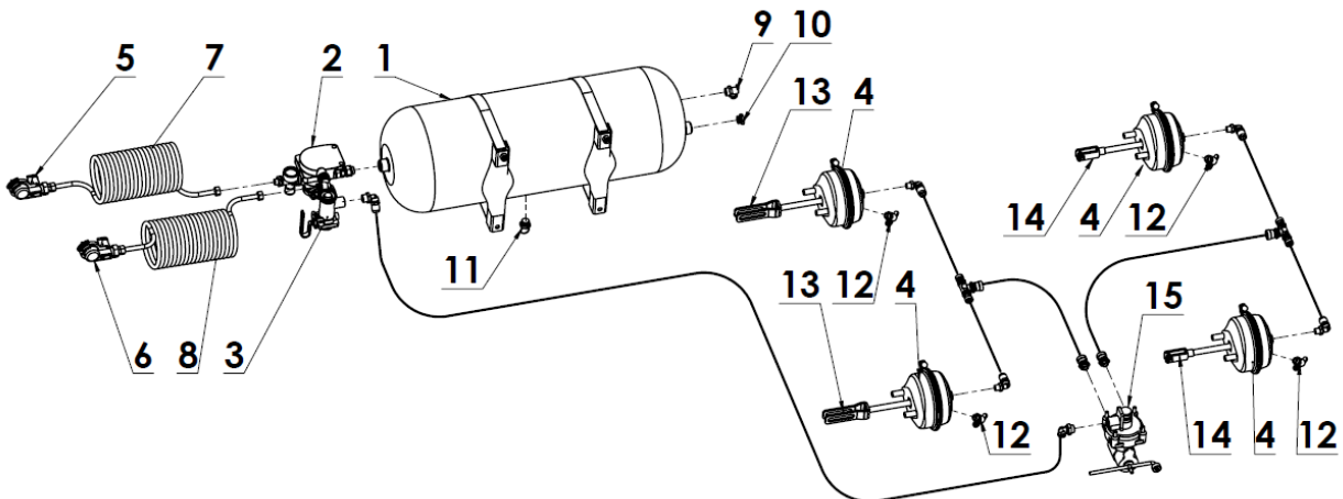
Rysunek 7. Instalacja hamulcowa pneumatyczna 2-przewodowa z zaworem ALB:
