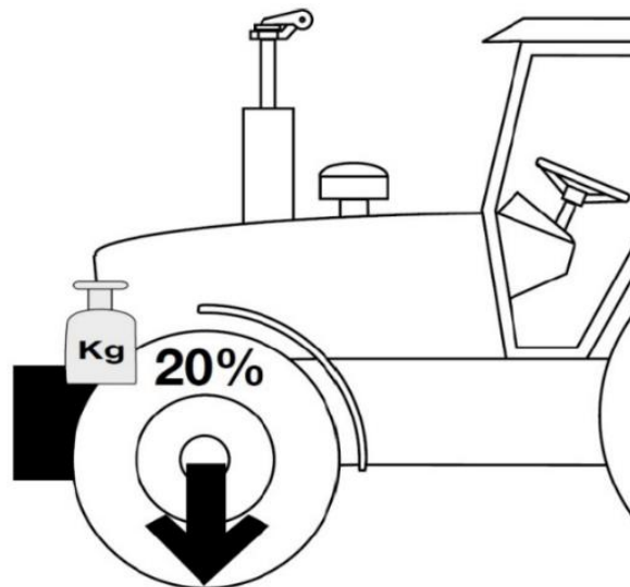
Rysunek 2. Minimalny nacisk na oś przednią ciągnika
