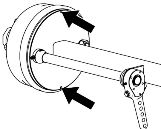
Rysunek 31. Kontrola zużycia okładzin hamulców
