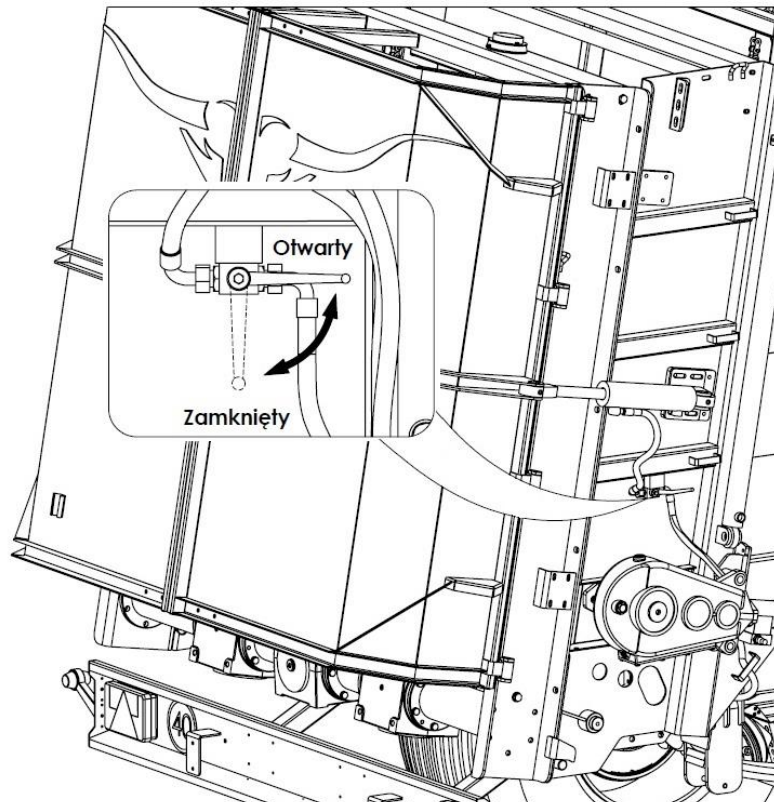
Rysunek 23. Zawór hydrauliczny blokujący osłonę adaptera
