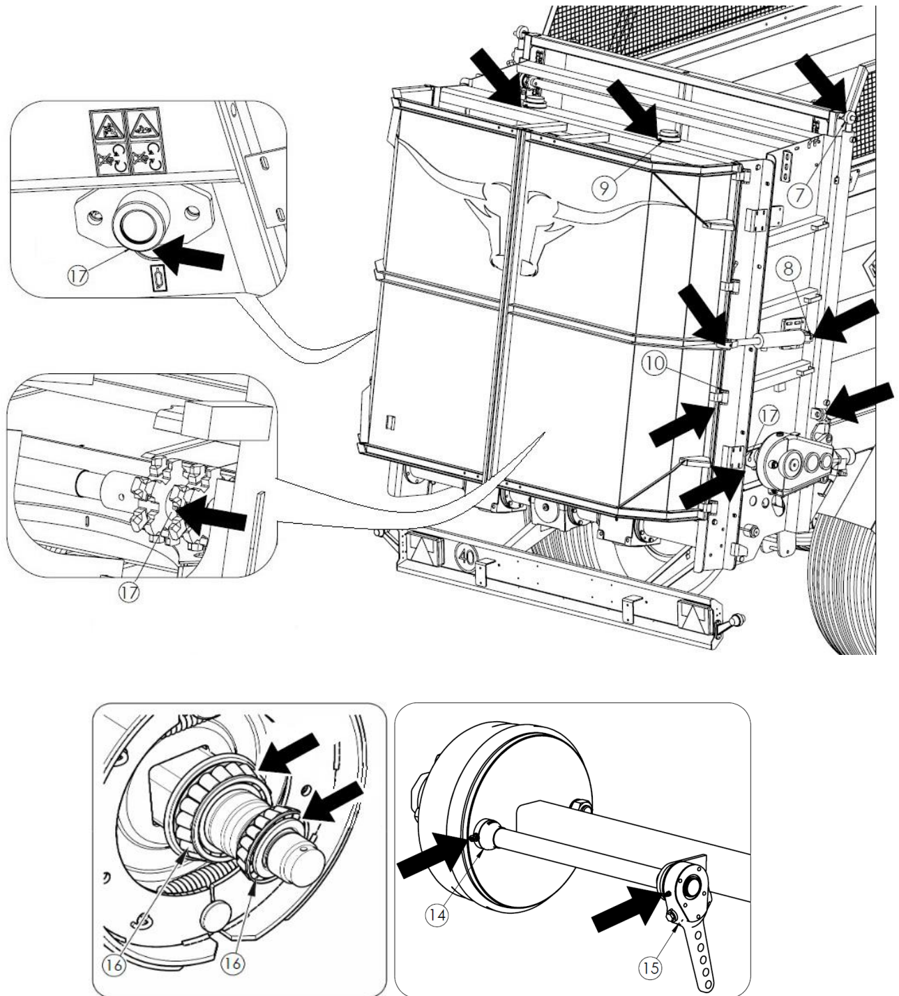
Rysunek 31. Punkty smarne rozrzutnika
