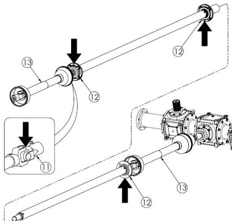
Rysunek 30. Punkty smarne rozrzutnika
