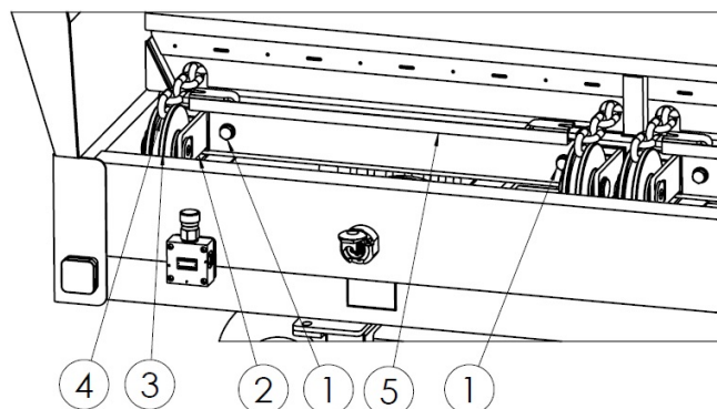
Rysunek 24. Napinanie łańcuchów przenośnika podłogowego 1 - śruba regulacyjna, 2 – suwak napinacza, 3- rolka napinacza, 4 – łańcuch przenośnika, 5 – listwa przenośnika
