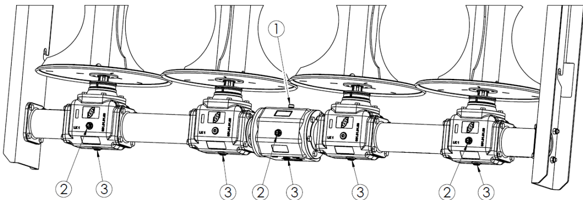
Rysunek 29. Punkty kontroli poziomu oleju przekładni adaptera pionowego 4-wirnikowego 1 - wlew oleju (odpowietrznik), 2 - wznik poziomu oleju, 3 - korki spustowe
