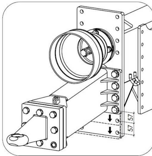
Rysunek 21. Regulacja wysokości zaczepu
