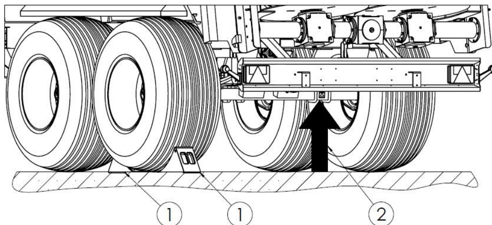
Rysunek 40. Punkty przyłożenia podnośników 1 - kliny, 2 - podnośnik
