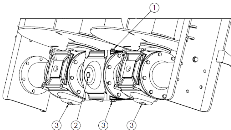
Rysunek 28. Punkty kontroli poziomu oleju przekładni adaptera pionowego 2-wirnikowego i adaptera trczowo-poziomego 2-wirnikowego 1 - wlew oleju (odpowietrznik), 2 - wznik poziomu oleju, 3 - korki spustowe
