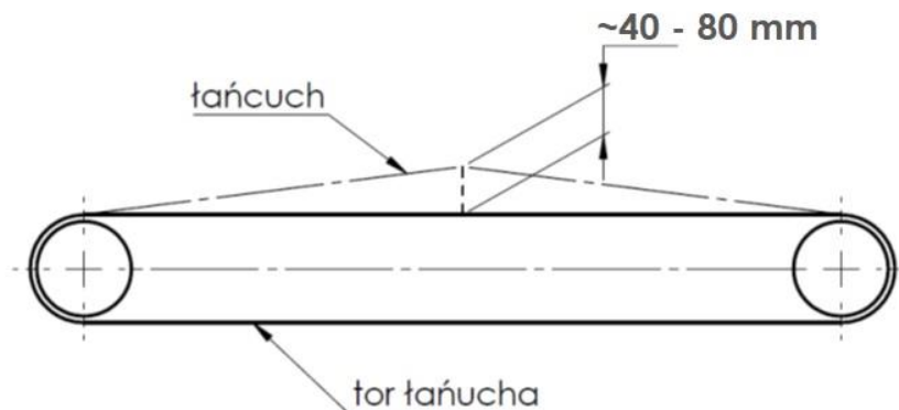
Rysunek 25. Sprawdzenie naciągu łańcucha w rozrzutniku
