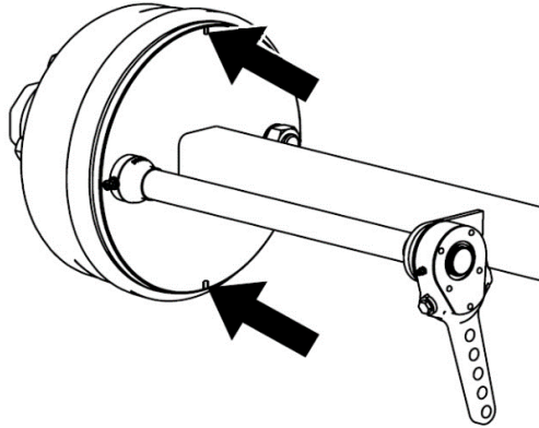
Rysunek 38. Kontrola zużycia okładzin hamulców
