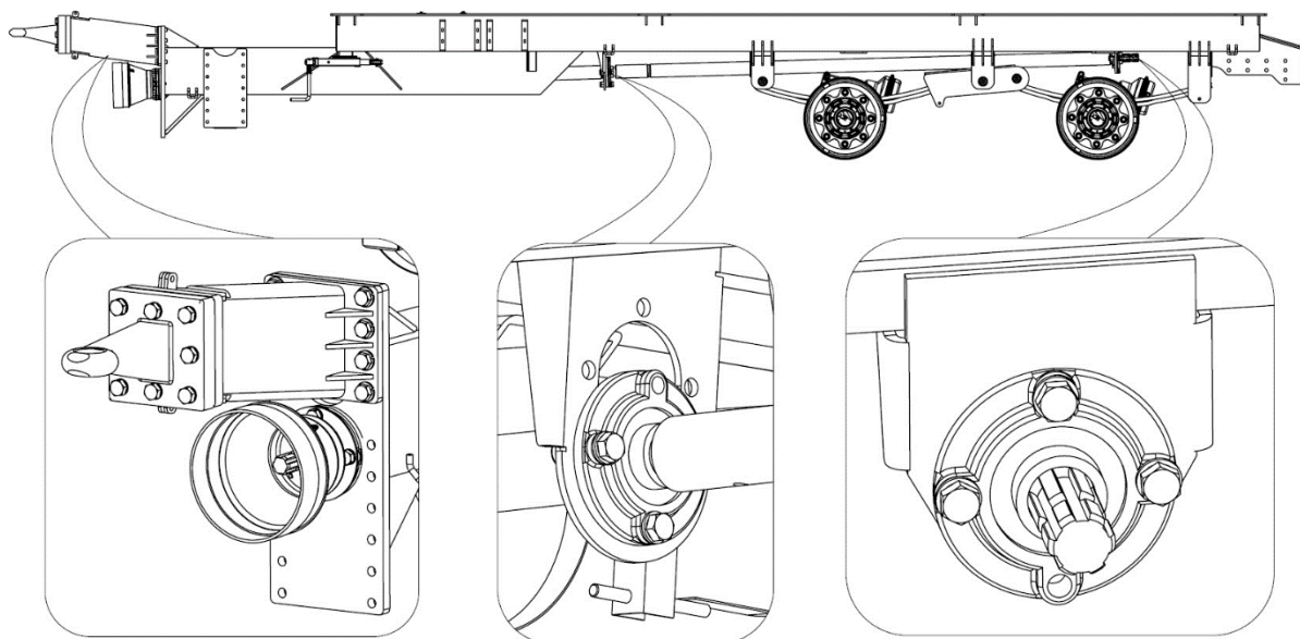
Rysunek 19. Położenie zacze­pu przystosowanego do łączenia z dolnym zaczepem ciągnika
