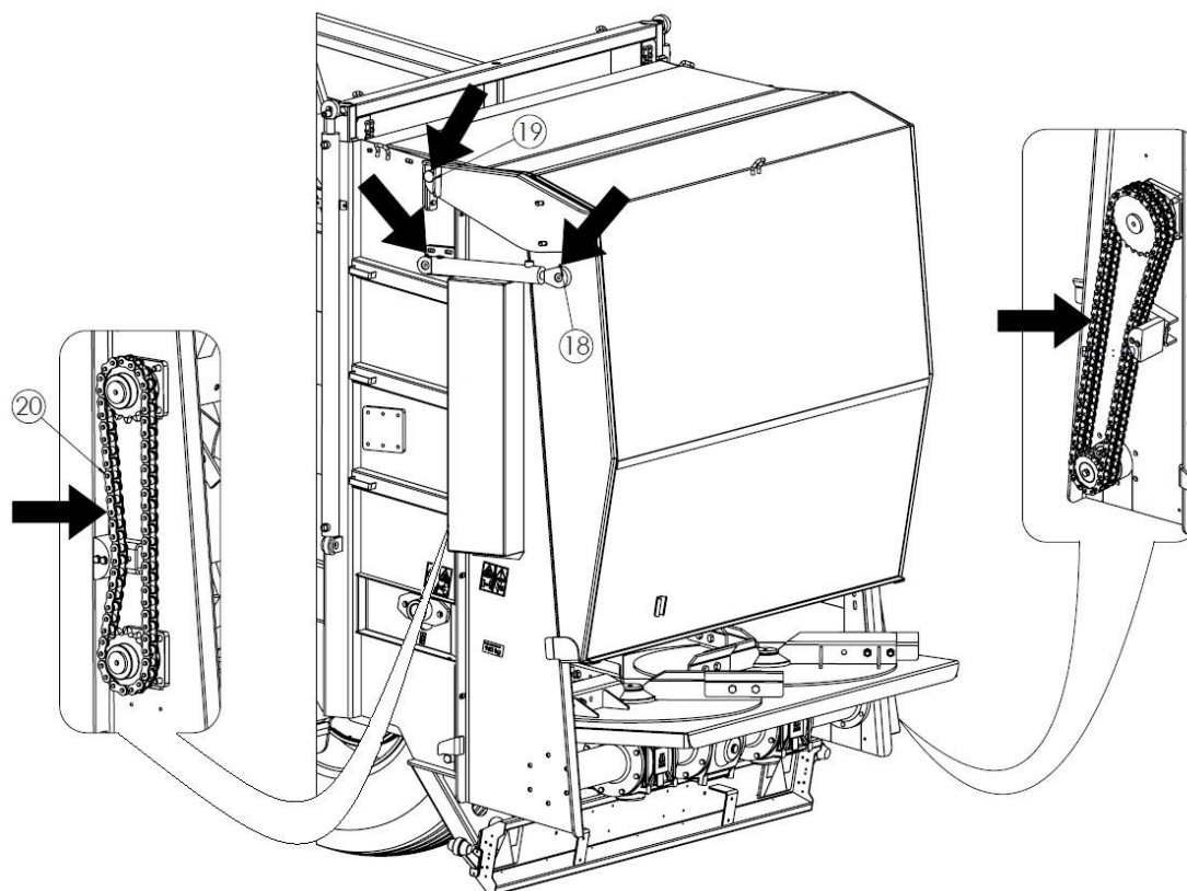
Rysunek 32. Punkty smarne rozrzutnika (adapter tarczowo-poziomy 2-wirnikowy)
