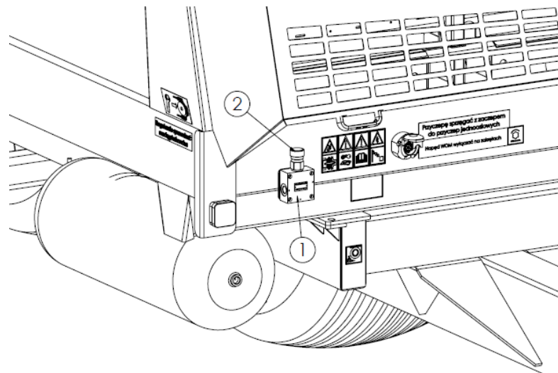
Rysunek 22. Regulacja prędkości przesuwu przenośnika podłogowego 1 - regulator przepływu oleju, 2 - pokrętło regulatora
