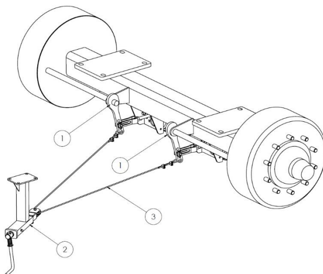
Rysunek 11. Hamulec postojowy: 1 - dźwignia rozpieracza, 2 - naciąg hamulca, 3 - linka stalowa L=5000 mm
