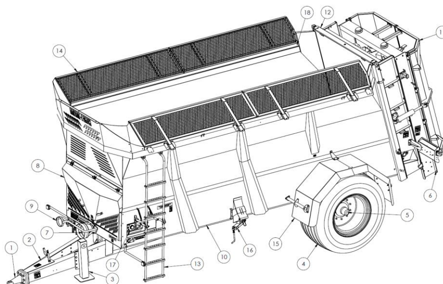
Rysunek 5. Ogólna budowa rozrzutnika obornika
