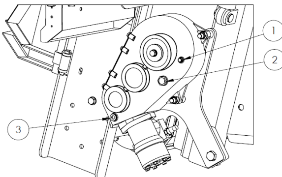
Rysunek 18. Punkty kontroli poziomu oleju przekładni przenośnika podłogowego. 1 - wlew oleju (odpowietrznik), 2 - wziernik poziomu oleju, 3 - korek spustowy
