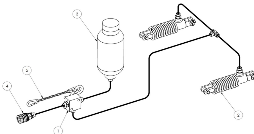
Rysunek 9. Instalacja hamulcowa hydrauliczna 1-przewodowa
