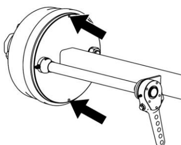
Rysunek 26. Kontrola zużycia okładzin hamulców
