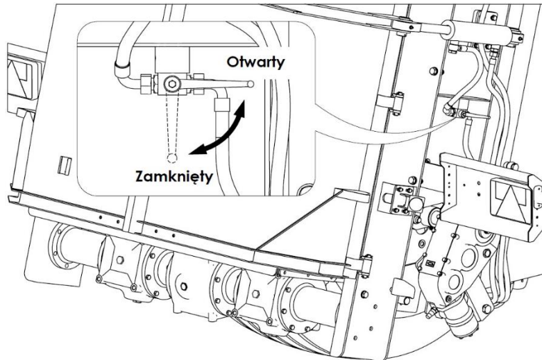
Rysunek 16. Zawór hydrauliczny blokujący osłonę adaptera
