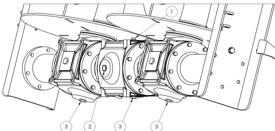
Rysunek 19. Punkty kontroli poziomu oleju przekładni adaptera. 1 - wlew oleju (odpowietrznik), 2 - wziernik poziomu oleju, 3 - korki spustowe
