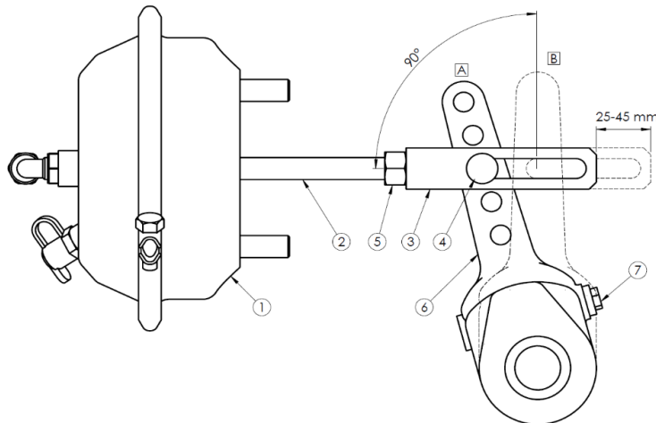
Rysunek 27. Regulacja hamulca zasadniczego
