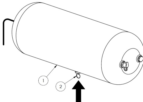
Rysunek 24. Odwadnianie zbiornika powietrza: 1 - zbiornik powietrza, 2 - zawór odwadniający
