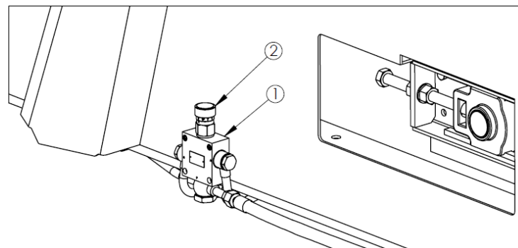
Rysunek 15. Regulacja prędkości przesuwu przenośnika podłogowego 1 - regulator przepływu oleju, 2 - pokrętko regulatora
