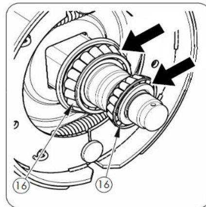
Rysunek 21. Punkty smarne rozrzutnika
