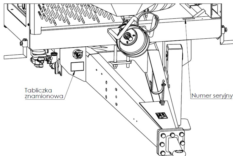
Rysunek 2. Położenie tabliczki znamionowej i numeru seryjnego
