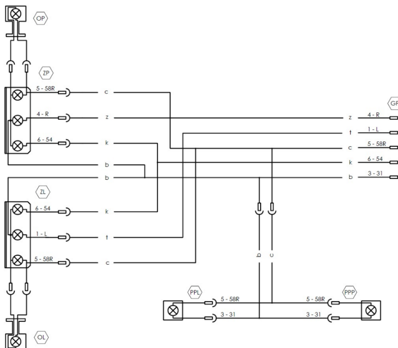
Rysunek 12. Schemat instalacji elektrycznej
