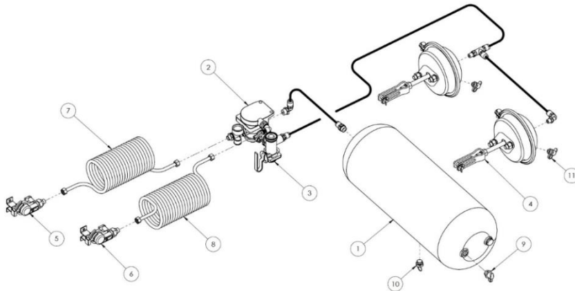
Rysunek 7. Instalacja hamulcowa pneumatyczna 2-przewodowa
