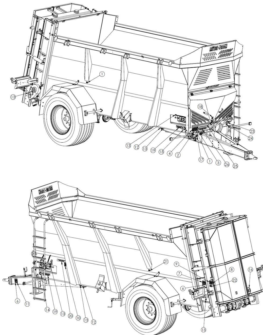
Rysunek 4. Rozmieszczenie naklejek ostrzegawczych i informacyjnych
