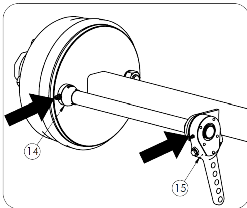
Rysunek 21. Punkty smarne rozrzutnika
