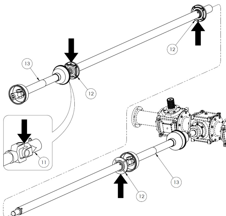
Rysunek 20. Punkty smarne rozrzutnika
