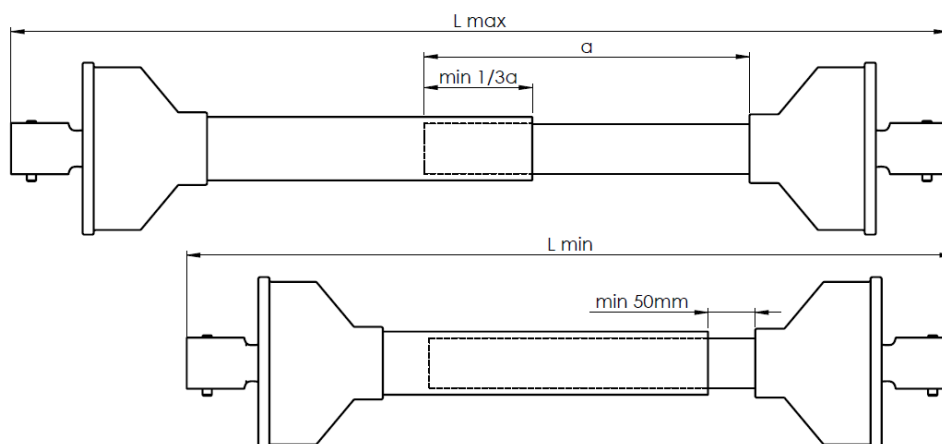
Rysunek 14. Dopasowanie długości wału przy podłączeniu rozrzutnika do ciągnika
