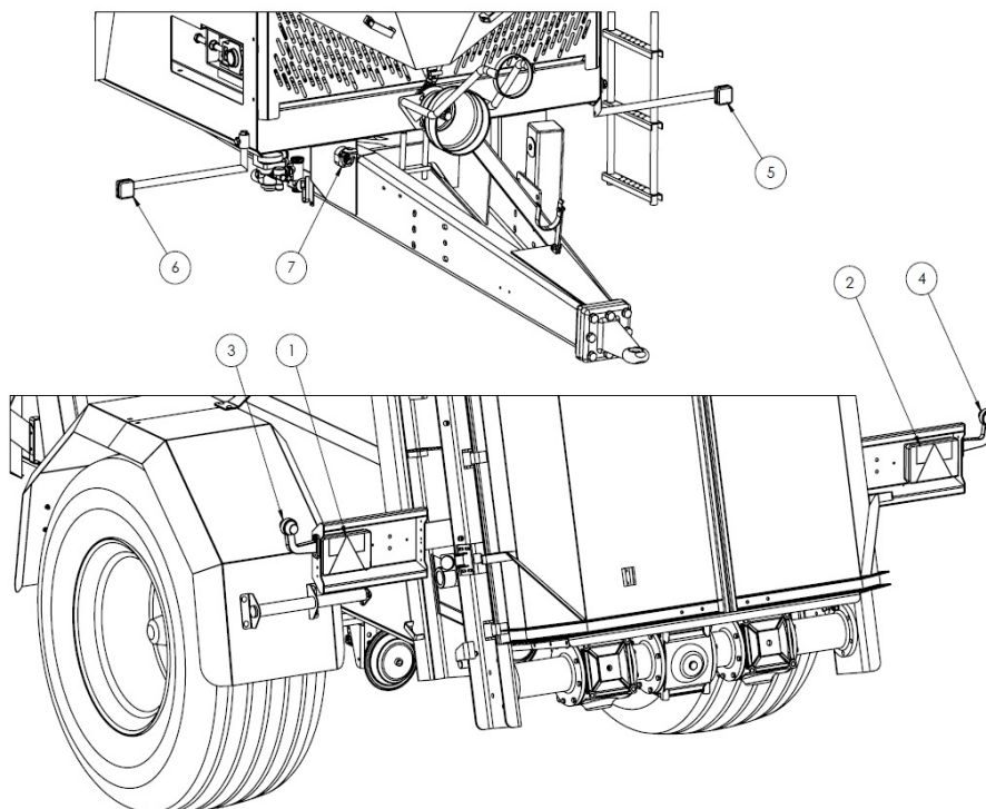
Rysunek 13. Rozmieszczenie elementów instalacji elektrycznej
