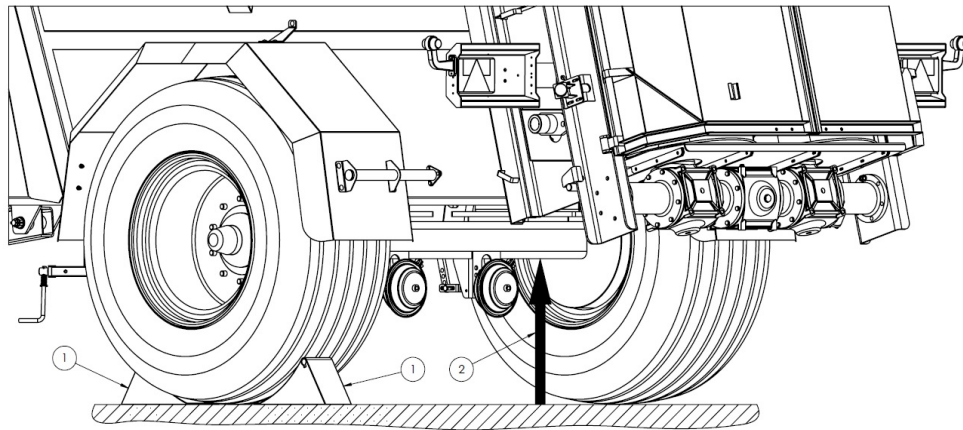
Rysunek 28. Punkty przyłożenia podnośników: 1 - kliny, 2 - podnośnik
