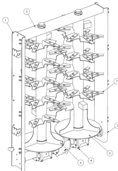
Rysunek 6. Adapter pionowy 2-wirnikowy
