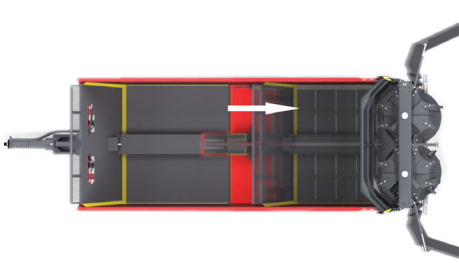
System zsuwający nadający się również do ciężkich ładunków
