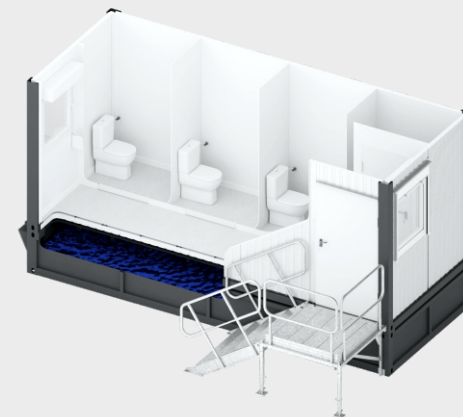
Przykładowy kontener sanitarny. Widok wewnętrzny
